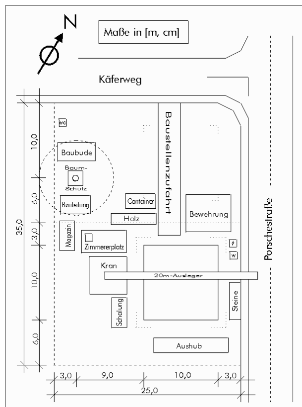
Baustelleneinrichtungsplan
