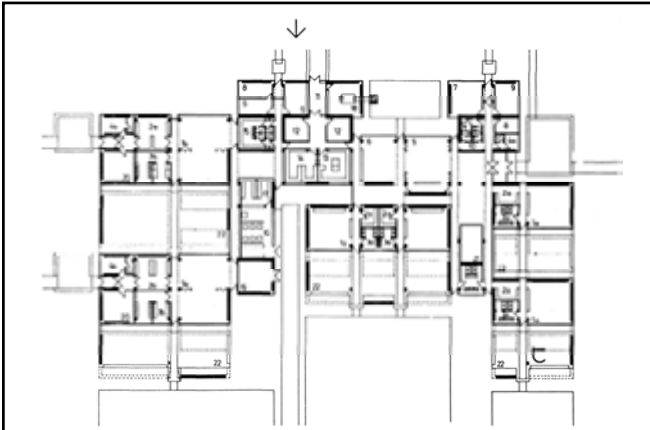
Ivan Crnković, 1975., Dječji vrtić, Samobor
