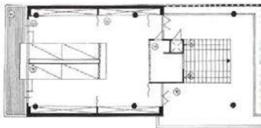
Nikola Dobrović, 1938., Vila Rusalka (Pallavicini), Ivana Matijaševića 2, Boninovo, Dubrovnik
