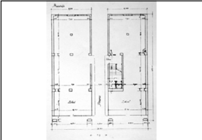
Drago Ibler, 1930., Stambeno-poslovna zgrada Wellisch, Martićeva 13, Zagreb
