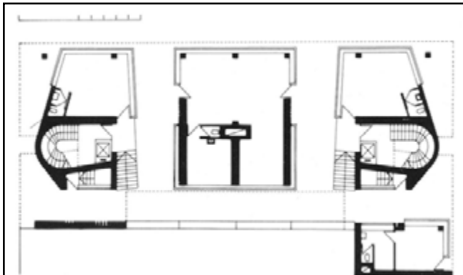
Alfred Albini, 1954.god., Stambeno-poslovna zgrada, Dalmatinskog Sabora 3 i 4, Zadar
