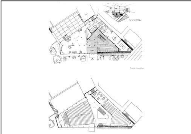
Ivan Vitić, 1947.-1961., Dom JNA, Poljana, Sibenik
