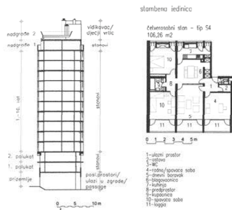
Frano Gotovac, 1970., Višestambena zgrada (Kineski zid), Rendićeva ulica, Spinut, Splat
