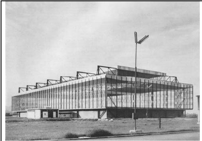
1957., Božidar Rašica, Paviljon Mašinogradnja, Zagrebački velesajam, Zagreb
