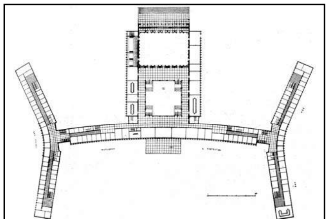
1947., Vladimir Potočnjak / Zlatko Neumann / Antun Ulrich / Dragica Perak, Predsjedništvo vlade FNRJ, Beograd
