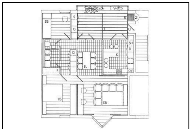
1983.-1991., Nikola Bašić, Stambeni blok 9 A, Bili brig, Zadar
