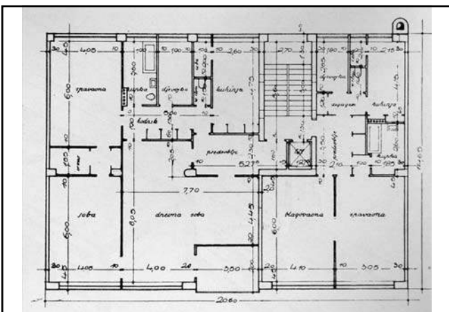
1930., Drago Ibler, Stambeno-poslovna zgrada Wellisch, Zagreb
