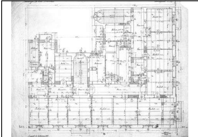
1914., Viktor Kovačić, Stambena zgrada (Kuća Frank), Zagreb
