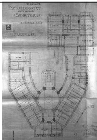
1910., Ignjat Fischer, Sanatorij dr. Jokovića, Zagreb
