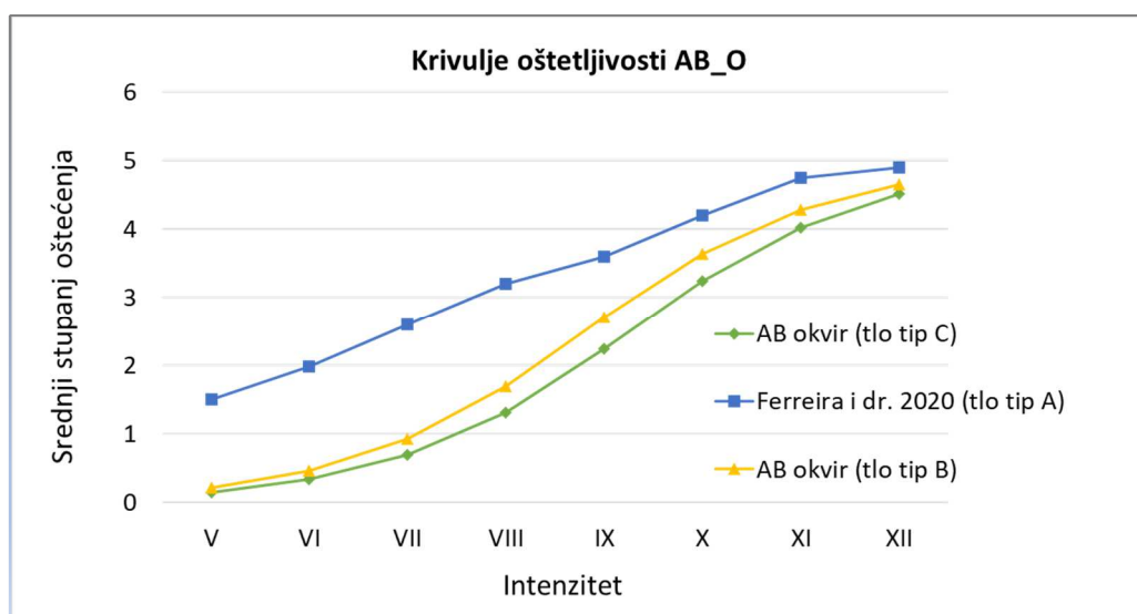
Slika 5.16 Krivulje oštetljivosti na različitom temeljnom tlu
