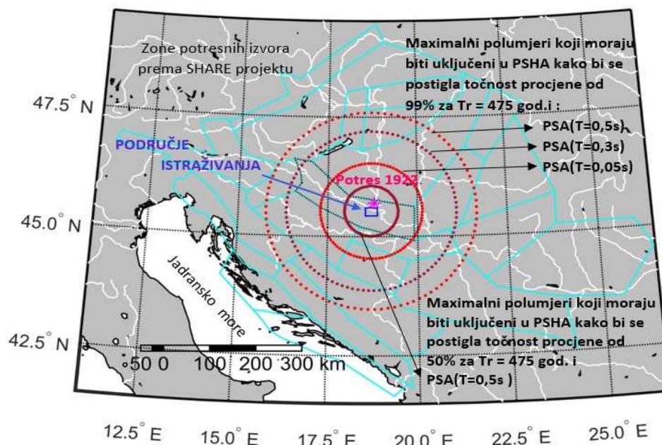
Slika 3.28 Maksimalni polumjeri za područje istraživanja koji moraju biti uključene u PSHA proračune vertikalnih vrijednosti spektralnih amplituda kako bi se postigla točnost ukupne procjene od: 99 % za T_r 475 god. za PSA(T = 0,5 s) = 229 km, PSA(T = 0,3 s) = 185 km, PSA(T = 0,05 s) = 111 km 50 % za T_r 475 god. i za PSA(T = 0,5 s) = 58 km (Bulajić i dr. 2021b)
