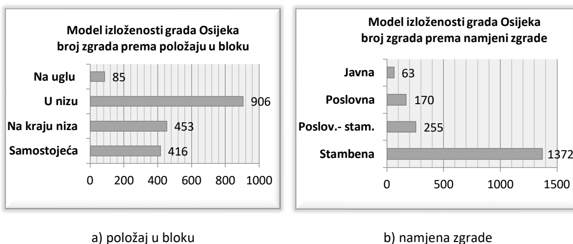
Slika 4.21 Brojnost zgrada prema nekonstrukcijskim karakteristikama
