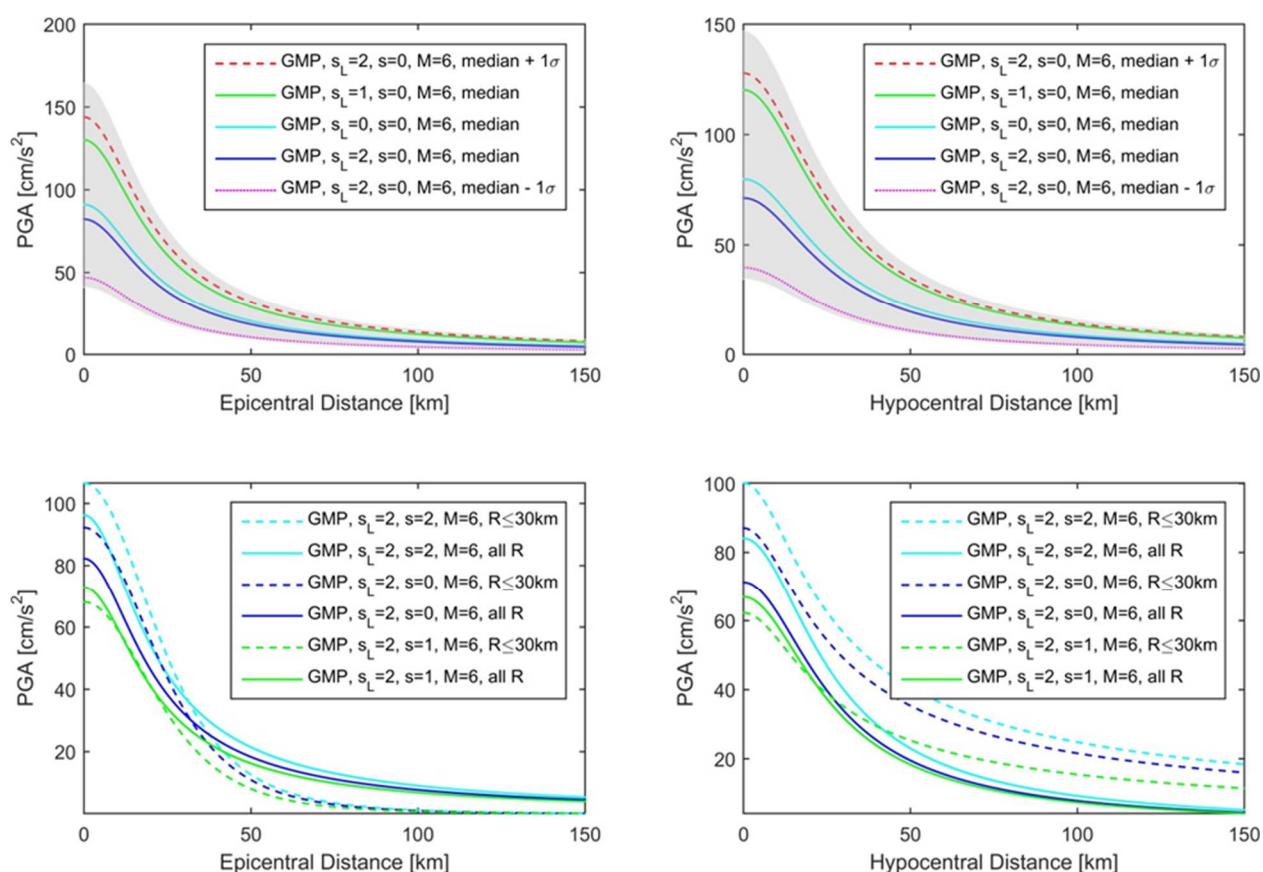
Slika 3.17 Empirijske atenuacijske krivulje vertikalnih vrijednosti PGA za različite lokalne i duboke geološke uvjete tla (vidi tablicu 3.8), proračunate jednadžbama (3.18) do (3.21) (Bulajić i dr. 2022a)
