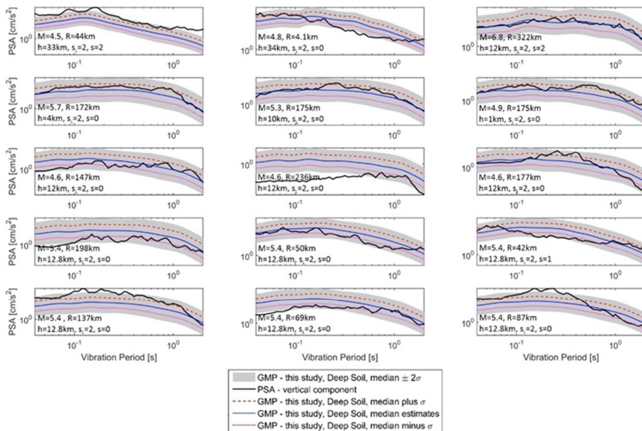
Slika 3.24 Odnos između regionalnih vertikalnih spektara pseudoubznanja na slojevima lokalnog temeljnog tla ( s_L = 2 ) i empirijskih predviđanja definiranih jednačbom (3.23) (Bulajić i dr. 2021b)
