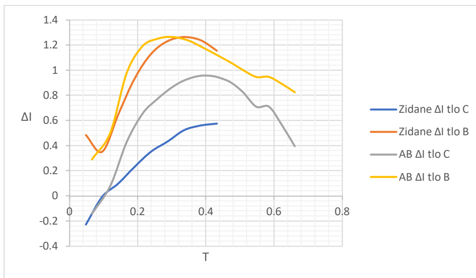
Slika 5.6 Grafička usporedba prirasta intenziteta \Delta I_{s,n} za zidane i armiranobetonske zgrade
