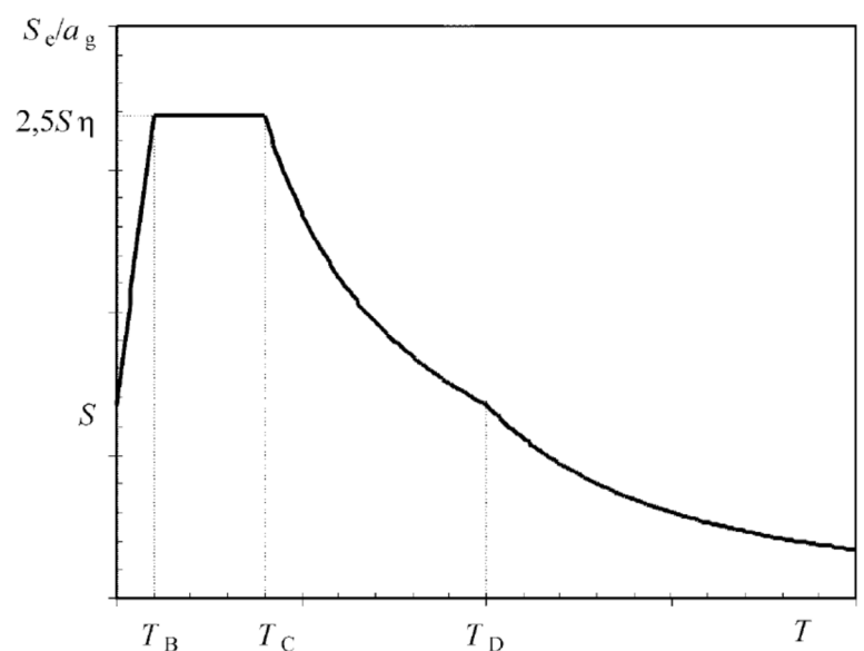
Slika 3.11 Elastični spektar odziva tip 1 (HRN EN 1998-1:2011/NA:2011)
