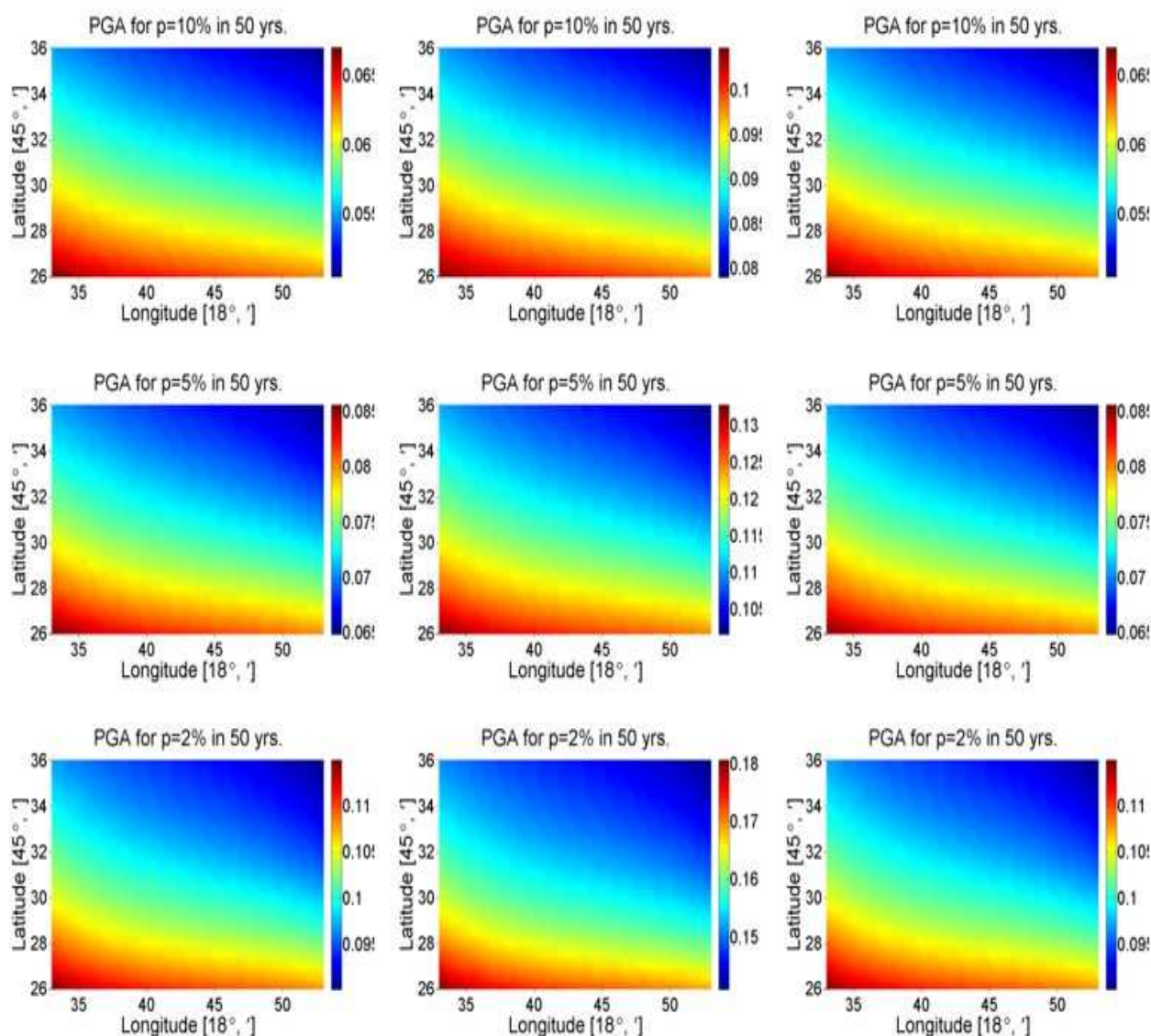
Slika 3.8 Vrijednosti PGA za stijenu (lijevo), plitko aluvijalno tlo (sredina) i duboko aluvijalno tlo (desno), dobivene probabilističkim proračunom potresne opasnosti za područje istraživanja, upotrebom atenuacijske jednadžbe Sabetta i Pugliese (1996.), za vjerojatnost 10 % u 50 godina (tj. povratno razdoblje od 475 godina), 5 % u 50 godina (povratno razdoblje od 975 godina) i 2 % u 50 godina (povratno razdoblje od 2475 godina)
