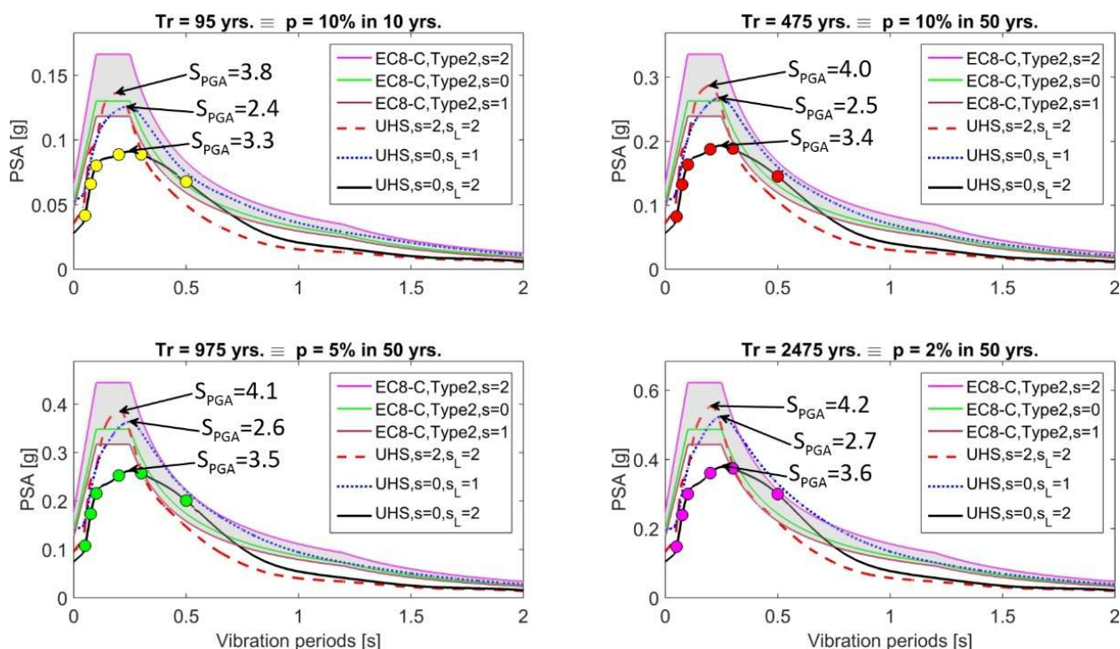
Slika 3.44 Usporedba spektara jednolike opasnosti iz horizontalnih amplituda PSA proračunatih za centralnu lokaciju područja istraživanja za četiri različite razine vjerojatnosti ponovljivosti sa spektrima Tip 2 prema HRN EN 1998:2011 (HRN EN 1998-1: 2011/NA:2011) za tlo tipa C (Bulajić i dr. 2021a)
