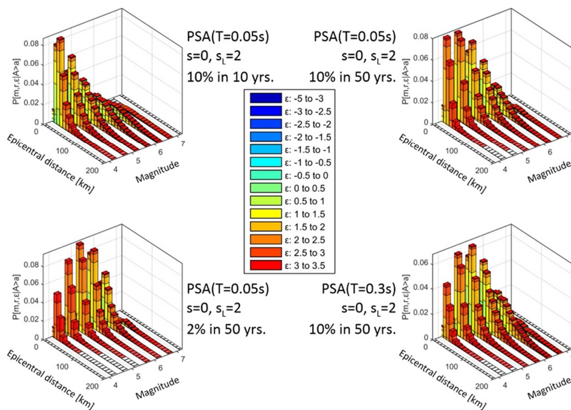
Slika 3.38 Primjeri rezultata razdvajanja potresne opasnosti horizontalnih PSA za centralnu lokaciju područja istraživanja (Bulajić i dr. 2021a)
