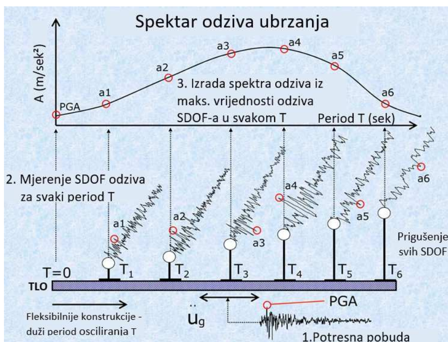
Slika 2.6 Generiranje spektra odziva ubrzanja
