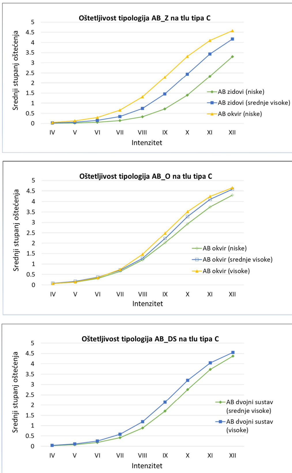
Slika 5.14 Srednji stupanj oštećenja tipologija armiranobetonaskih zgrada
