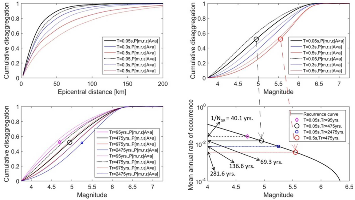
Slika 3.40 Primjeri razdvajanje doprinosa za udaljenost i magnitude, u kumulativnoj vrijednosti prekoračenja ( A > a ), odnosno dostizanja ( A = a ), horizontalnih spektralnih amplituda pseudoubznanja te krivulja ponovljivosti magnitude za područje potresnog izvora koji najviše doprinosi seizmičnosti za centralnu lokaciju područja istraživanja (Bulajić i dr. 2021a)
