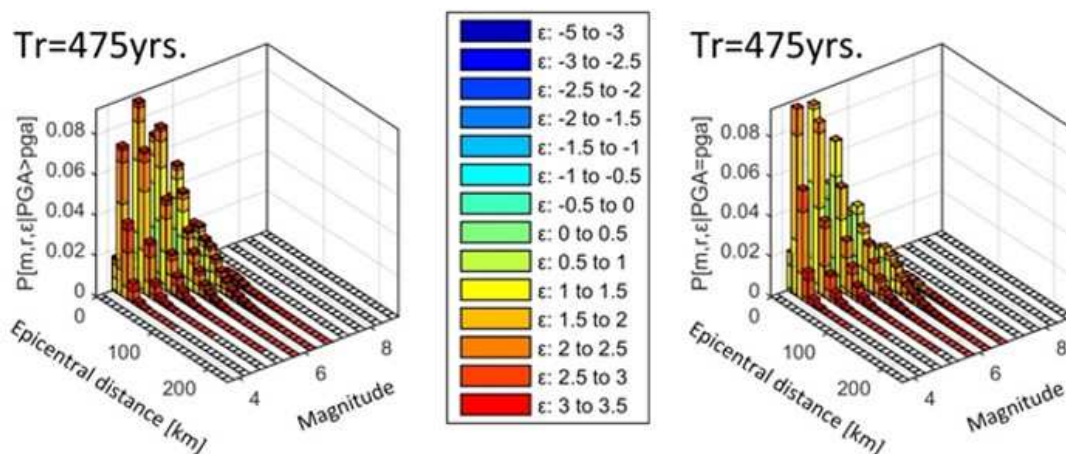
Slika 3.30 Razdvajanje potresne opasnosti za centralnu lokaciju područja istraživanja - vjerojatnosti doprinosa potresa različitih epicentralnih udaljenosti i magnituda u vrijednostima prekoračenja ( PGA > pga ) / dostizanja ( PGA = pga ) vertikalnih komponenata potresne opasnosti, za Tr = 475 godina Hrvatskoj (Bulajić i dr. 2022a)
