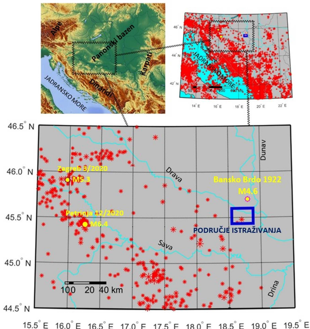
Slika 3.3 Područje istraživanja, smještaj te seizmološko-geološke karakteristike (prema Bulajić i dr. 2021a)
