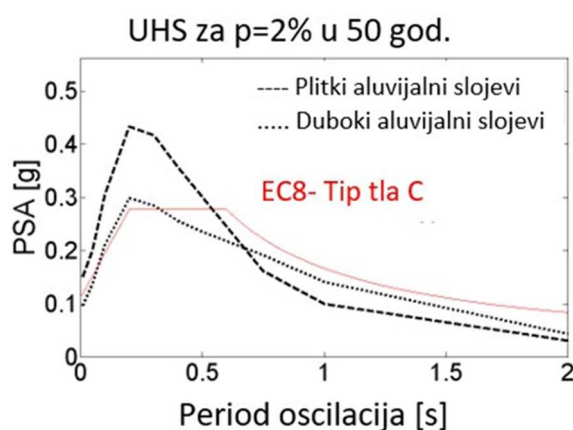
Slika 3.14 Spektri jednolike opasnosti za lokaciju 45,55 °N, 18,70 °E, proračunati uporabom atenuacijske jednadžbe Sabetta i Pugliese (1996.), za povratno razdoblje od 2475 godina uspoređeni s odgovarajućim spektrima HRN EN 1998-1:2011
