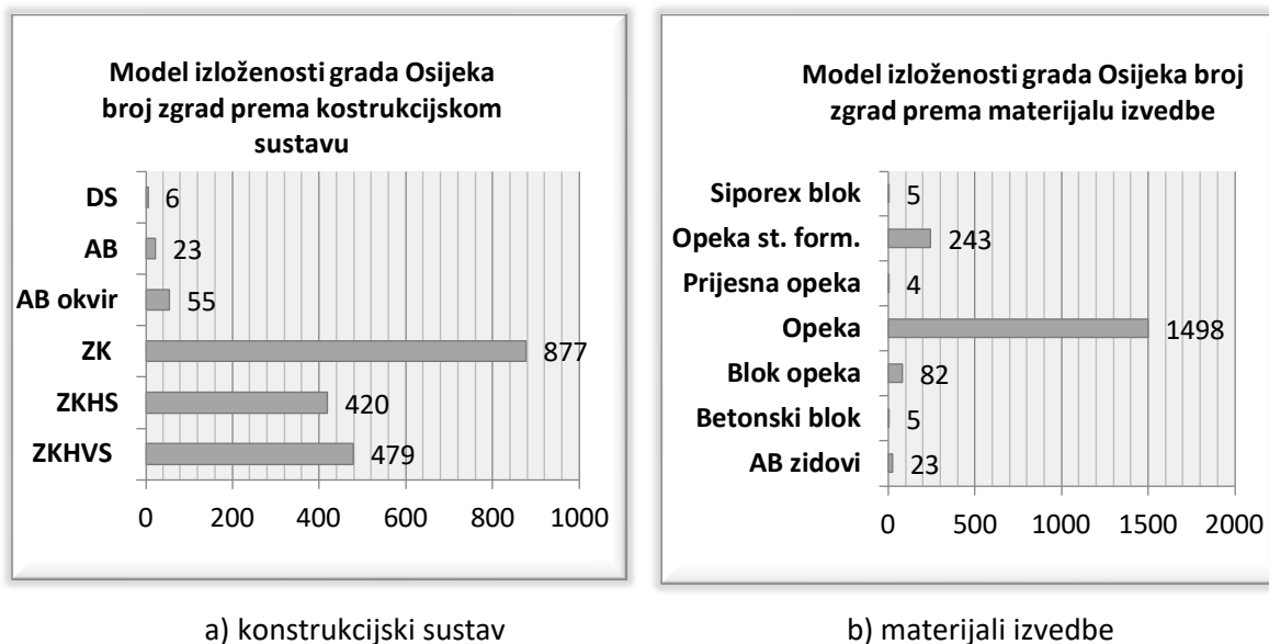
Slika 4.18 Brojnost zgrada prema konstrukcijskim karakteristikama i materijalima izvedbe
