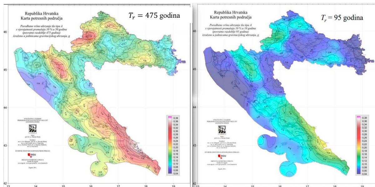
Slika 3.5 Karte potresne opasnosti Republike Hrvatske za povratna razdoblja 475 i 95 godina (Herak 2012)
