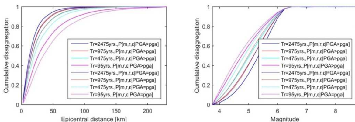
Slika 3.31 Razdvajanje doprinosa, epicentralnih udaljenosti i magnituda u kumulativnoj vrijednosti prekoračenja ( PGA > pga ) / dostizanja ( PGA = pga ) horizontalnih komponenata potresne opasnosti, za različita povratna razdoblja (Bulajić i dr. 2022b)
