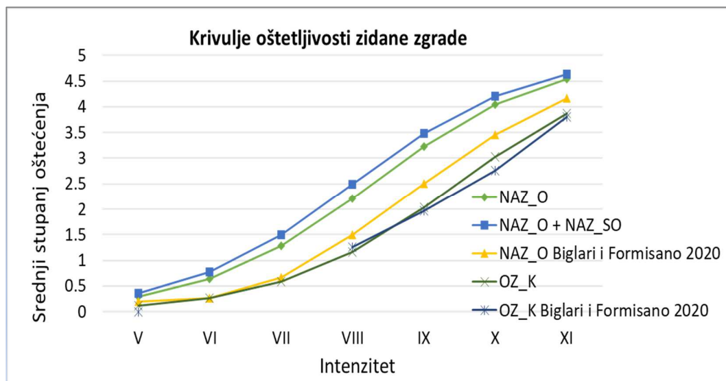
Slika 5.17 Krivulje oštećljivosti tipologija zidanih zgrada
