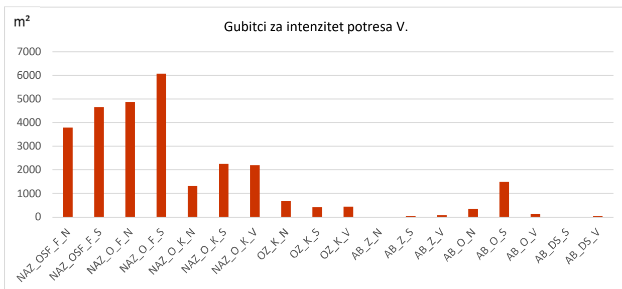
Slika 6.10 Gubitci za tipologije zgrade iz modela izloženosti grada Osijeka, za intenzitet V
