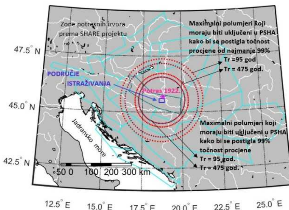
Slika 3.25 Maksimalni polumjeri za područje istraživanja koji moraju biti uključene u PSHA proračune horizontalnih vrijednosti PGA kako bi se postigla točnost ukupne procjene potresne opasnosti od: najmanje 99 % za Tr 95 god. = 205 km, za Tr 475 god. = 132,5 km točno 99 % za Tr 95 god. = 182,5 km, za Tr 475 god. = 115 km (Bulajić i dr. 2022b)
