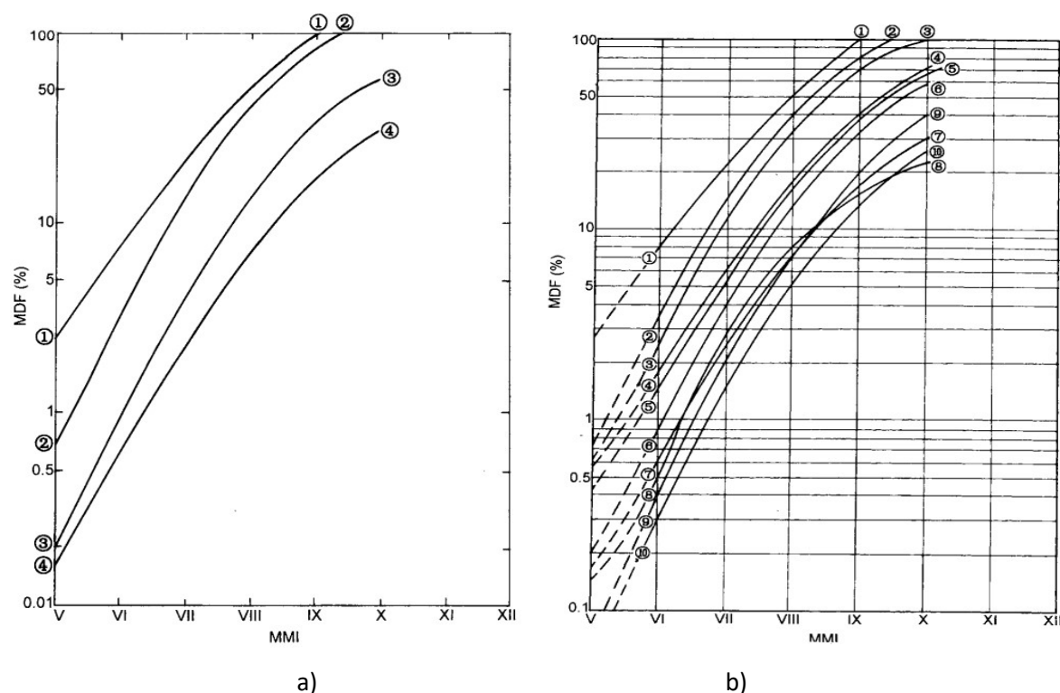
Slika 6.2 Krivulje oštećljivosti prema: a) Akkasu i Erdiku (1984.), b) Sauteru i Shahu (1978.)
