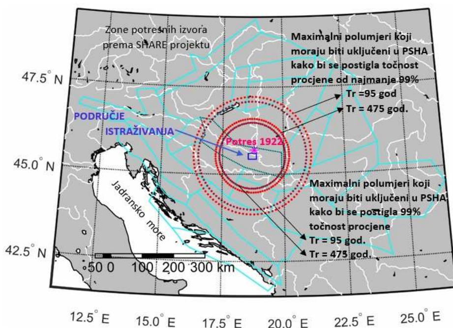
Slika 3.26 Maksimalni polumjeri za područje istraživanja koji moraju biti uključene u PSHA proračune vertikalnih vrijednosti PGA kako bi se postigla točnost ukupne procjene potresne opasnosti od: najmanje 99 % za T_r 95 god. = 187,5 km, za T_r 475 god. = 117,5 km točno 99 % za T_r 95 god. = 172,5 km, za T_r 475 god. = 105 km (Bulajić i dr. 2022a)
