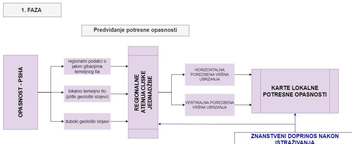
Slika 1.2 Shematski prikaz – predviđanje potresne opasnosti
