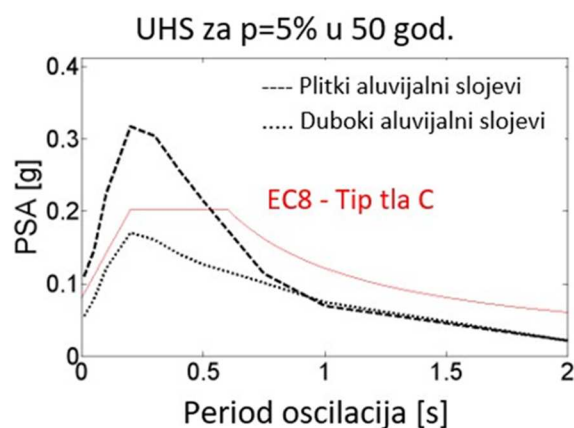
Slika 3.13 Spektri jednolike opasnosti za lokaciju 45,55 °N, 18,70 °E, proračunati uporabom atenuacijske jednadžbe Sabetta i Pugliese (1996.), za povratno razdoblje od 975 godina uspoređeni s odgovarajućim spektrima HRN EN 1998-1:2011
