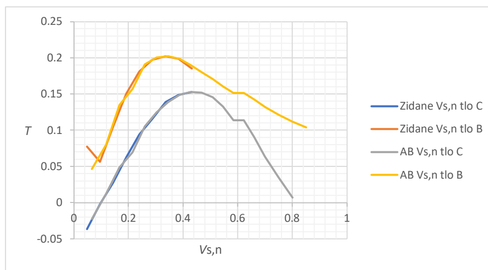
Slika 5.7 Raspodjela vrijednosti V_{s,n} za zidane i armiranobetonske zgrade
