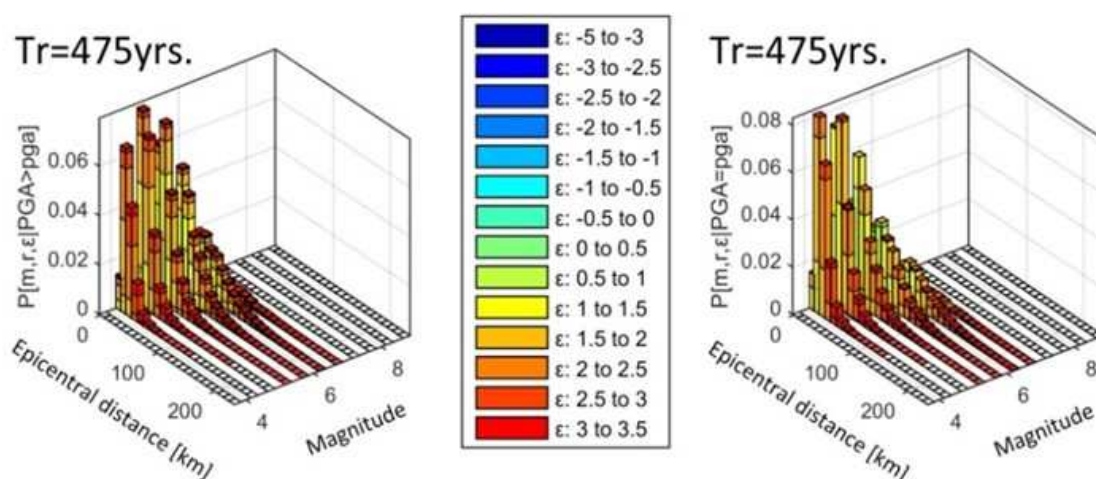
Slika 3.29 Razdvajanje potresne opasnosti za centralnu lokaciju područja istraživanja - vjerojatnosti doprinosa potresa različitih epicentralnih udaljenosti i magnituda u vrijednostima prekoračenja ( PGA > pga ) / dostizanja ( PGA = pga ) horizontalnih komponenta potresne opasnosti, za T_r = 475 godina (Bulajić i dr. 2022b)
