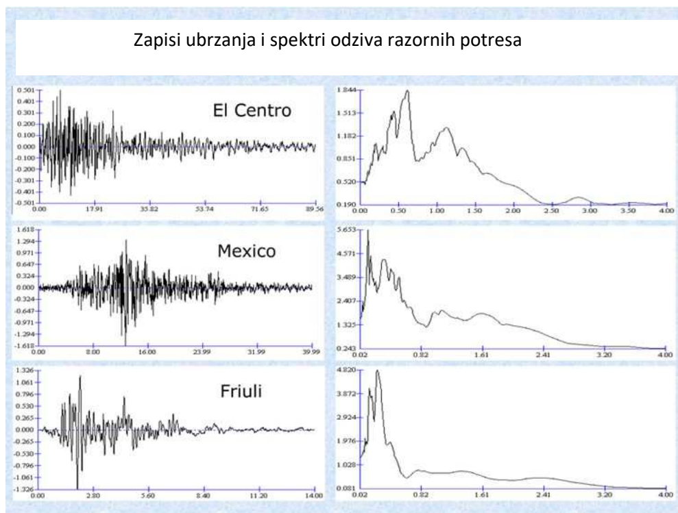
Slika 2.5 Zapisi potresa i spektri odziva ubrzanja za potrese koji su pogodili El Centro, Mexico City i Friuli
