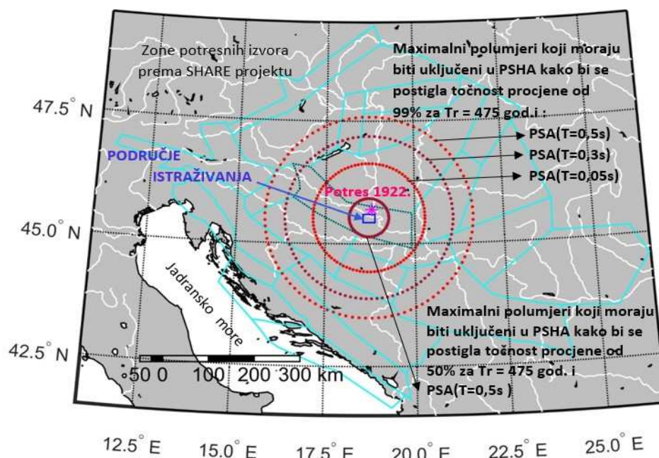
Slika 3.27 Maksimalni polumjeri za područje istraživanja koji moraju biti uključene u PSHA proračune horizontalnih vrijednosti spektralnih amplituda kako bi se postigla točnost ukupne procjene od: 99 % za T_r 475 god. za PSA(T = 0,5 s) = 228 km, PSA(T = 0,3 s) = 184 km, PSA(T = 0,05 s) = 123 km 50 % za T_r 475 god. i za PSA(T = 0,5 s) = 43 km (Bulajić i dr. 2021a)
