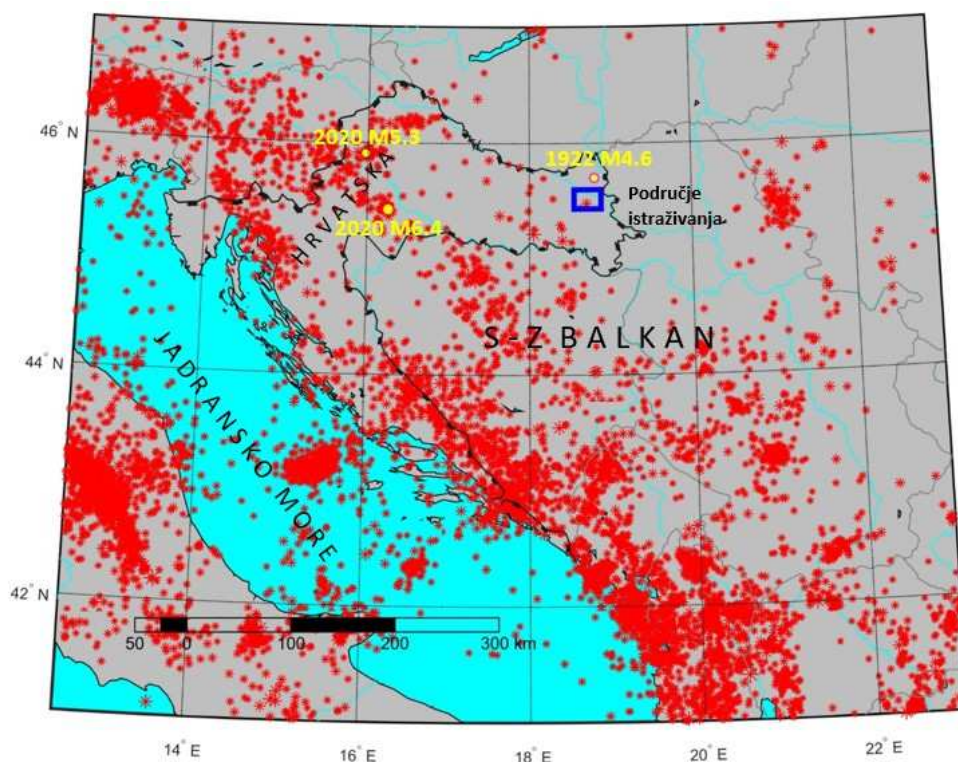
Slika 3.1 Epicentri regionalnih potresa zabilježeni između 1900. i travnja 2021. (USGS 2021), granice centralnog područja istraživanja (plavi okvir), epicentri: najvećeg povijesnog potres na području istraživanja (1922. s M = 4,6 ) te nedavnih (2020.-te ) potresa u Zagrebu ( M = 5,3 ) i Petrinji ( M = 6,4 ) (prema Pavić i dr. 2020a)
