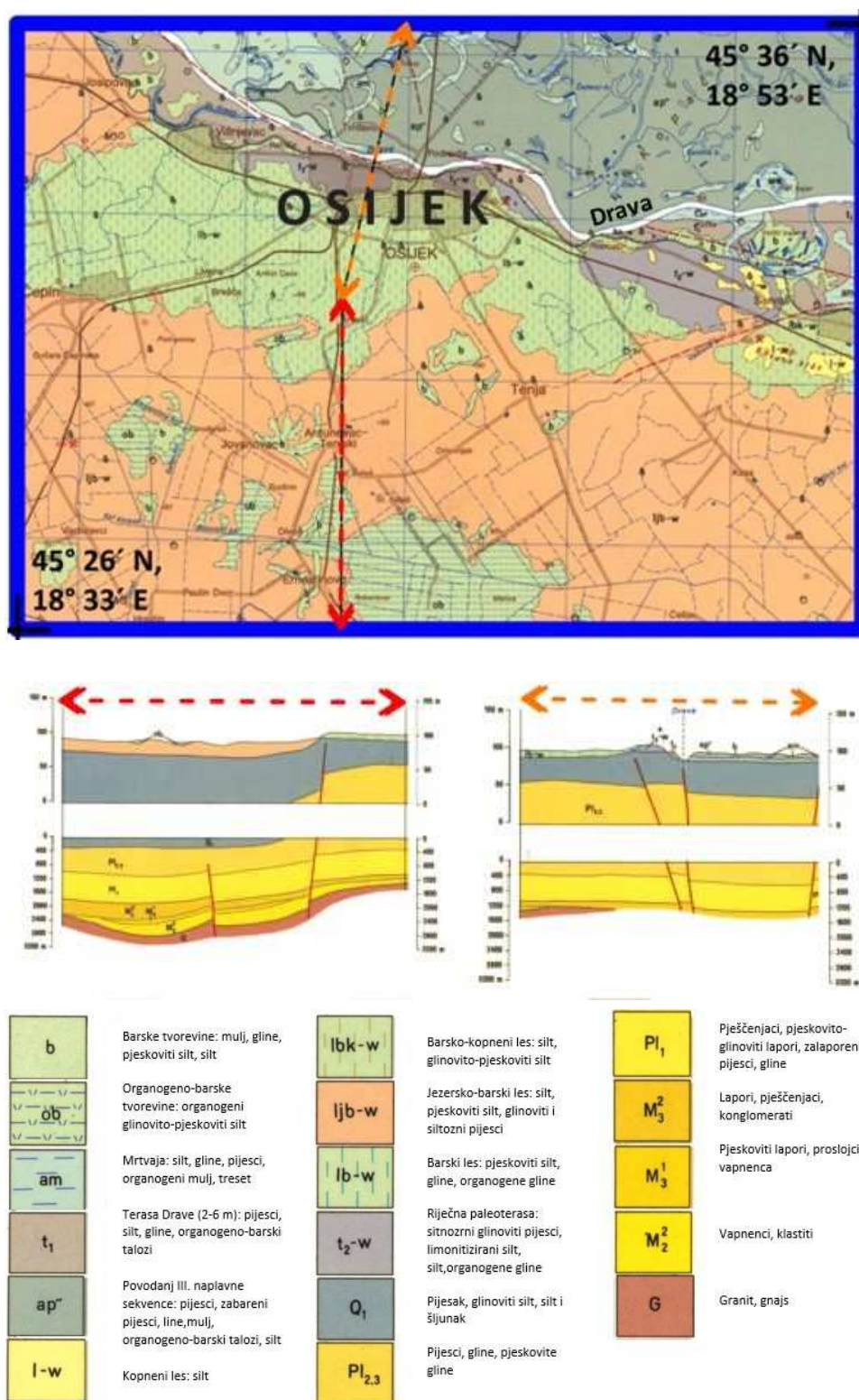
Slika 3.4 Uzdužni geološki profili područja istraživanja (prema Pikija i dr. 1991, Magaš i dr. 1987)
