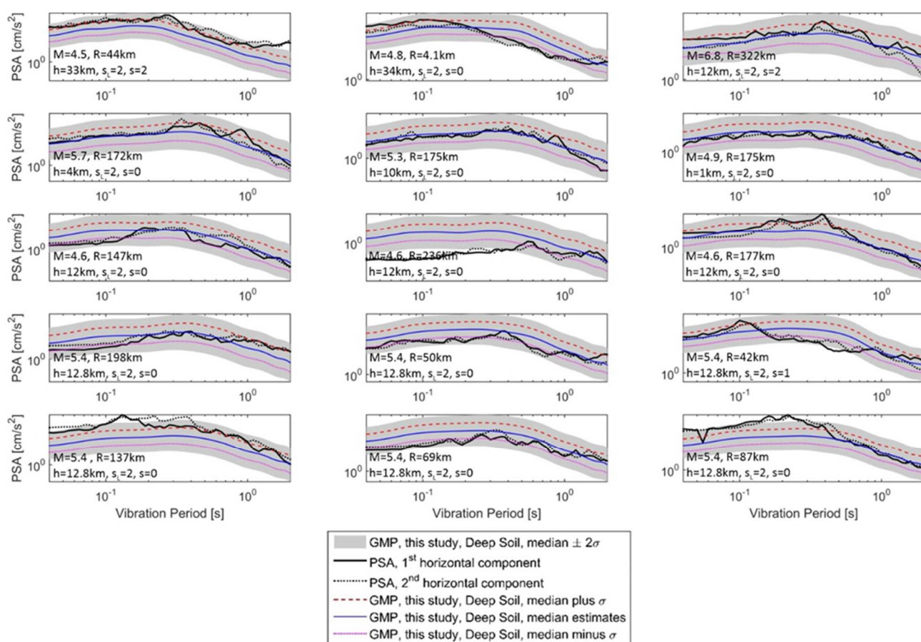
Slika 3.21 Usporedba između regionalnih horizontalnih spektara pseudoubiranja snimljenih na dubokim lokalnim tlima ( s_L = 2 ) i empirijska predviđanja jednadžbom (3.22) i koeficijentima iz tablice 3.10 (Bulajić i dr. 2021a)
