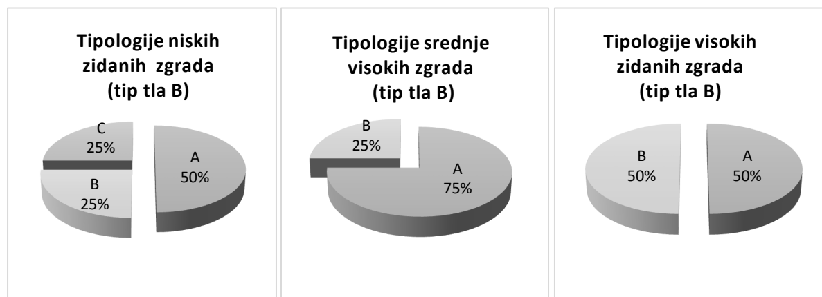
Slika 5.12 Postotak razreda oštetljivosti tipologija niskih zgrada razvrstanih prema visini (temeljno tlo tipa B)
