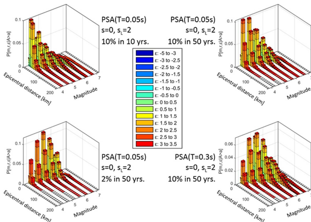
Slika 3.39 Primjeri rezultata razdvajanja potresne opasnosti vertikalnih PSA za centralnu lokaciju područja istraživanja (Bulajić i dr. 2021b)
