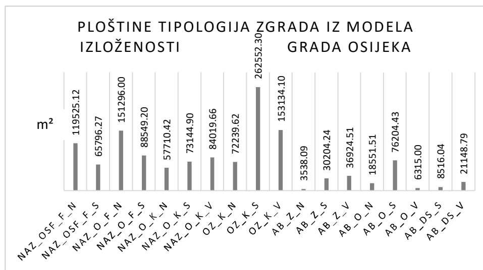
Slika 6.3 Ploštine tipologija zgrada iz modela izloženosti grada Osijeka
