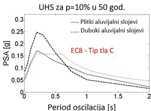
Slika 3.12 Spektri jednolike opasnosti za lokaciju 45,55 °N, 18,70 °E, proračunati uporabom atenuacijske jednadžbe Sabetta i Pugliese (1996.), za povratno razdoblje od 475 godina uspoređeni s odgovarajućim spektrima HRN EN 1998-1:2011
