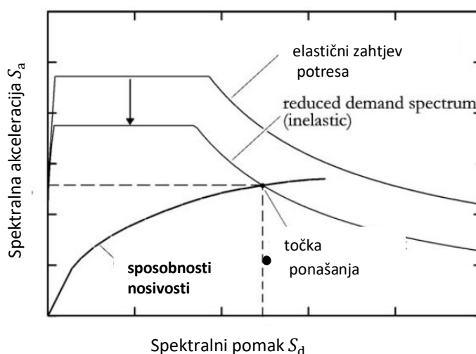
Slika 2.13 Grafički prikaz oštetljivost zgrade a) i b) pretvorba projektnog spektra odziva u S_a - S_d domenu, c) konstruiranje krivulje sposobnosti nosivosti
