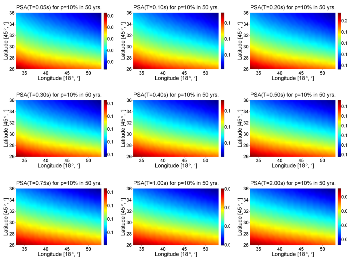
Slika 3.9 Vrijednosti niza spektralnih amplituda za duboko aluvijalno tlo, dobivene probabilističkim proračunom potresne opasnosti za područje istraživanja, upotrebom atenuacijskih jednadžbi za spektralne amplitude Sabetta i Pugliese (1996.), za vjerojatnost 10 % u 50 godina (povratno razdoblje od 475 godina)
