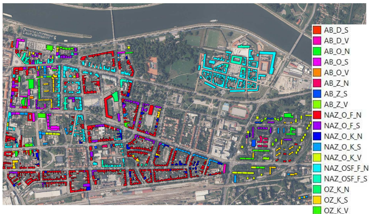
Slika 5.18 Raspodjela generiranih tipologija u modelu izloženosti grada Osijeka
