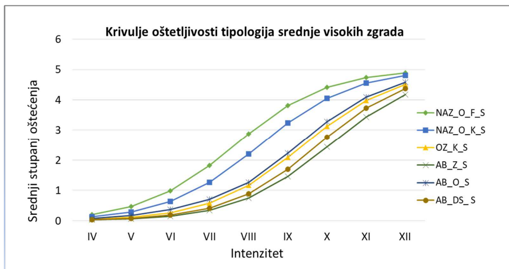
Slika 5.15 Usporedba krivulja oštećljivosti tipologija srednje visokih zgrada
