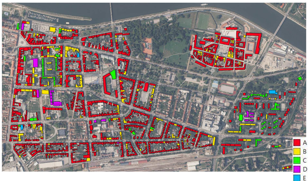
Slika 5.20 Raspodjela proračunatih razreda oštećljivosti za temeljno tlo tipa B u modelu izloženosti grada Osijeka
