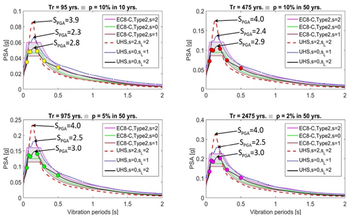
Slika 3.45 Usporedba spektara jednolike opasnosti iz vertikalnih amplituda PSA za centralnu lokaciju područja istraživanja za četiri različite razine vjerojatnosti ponovljivosti sa spektrima Tip 2 prema HRN EN 1998:2011 (HRN EN 1998-1: 2011/NA:2011) za tlo tipa C (Bulajić i dr. 2021b)
