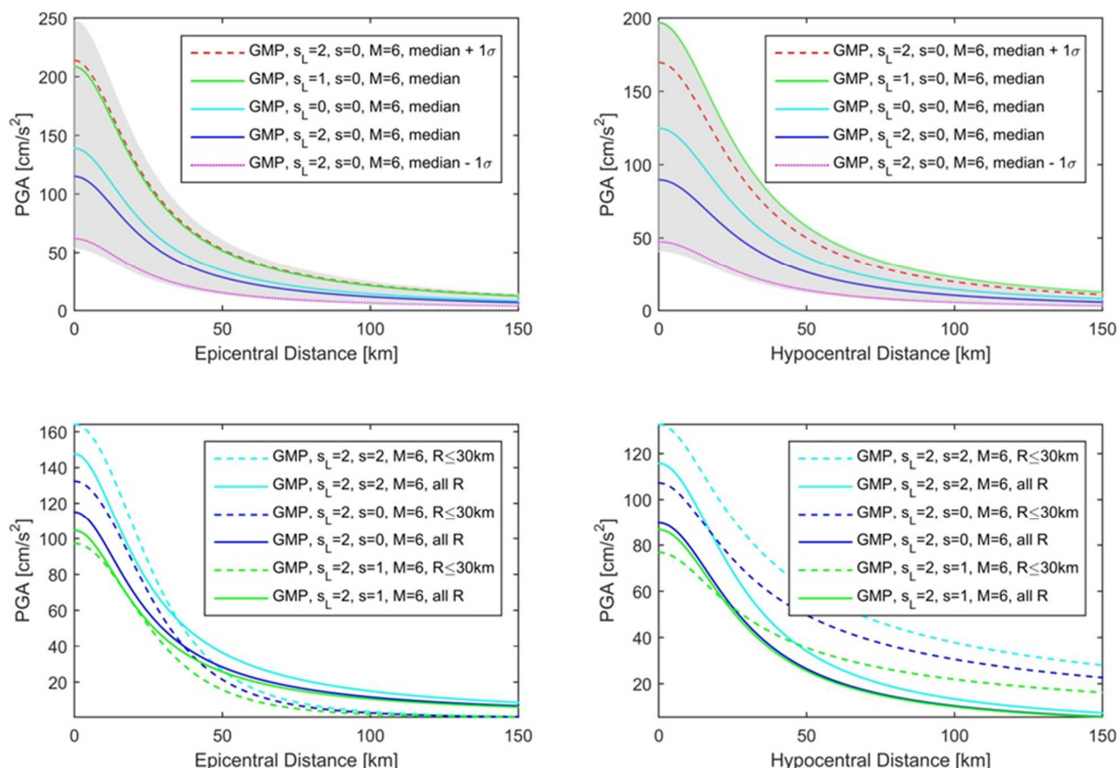
Slika 3.15 Empirijske atenuacijske krivulje horizontalnih vrijednosti PGA proračunate jednačbama (3.14) do (3.17), za različite uvjete lokalnog temeljnog tla i dubokih geoloških slojeva (Bulajić i dr. 2022b)
