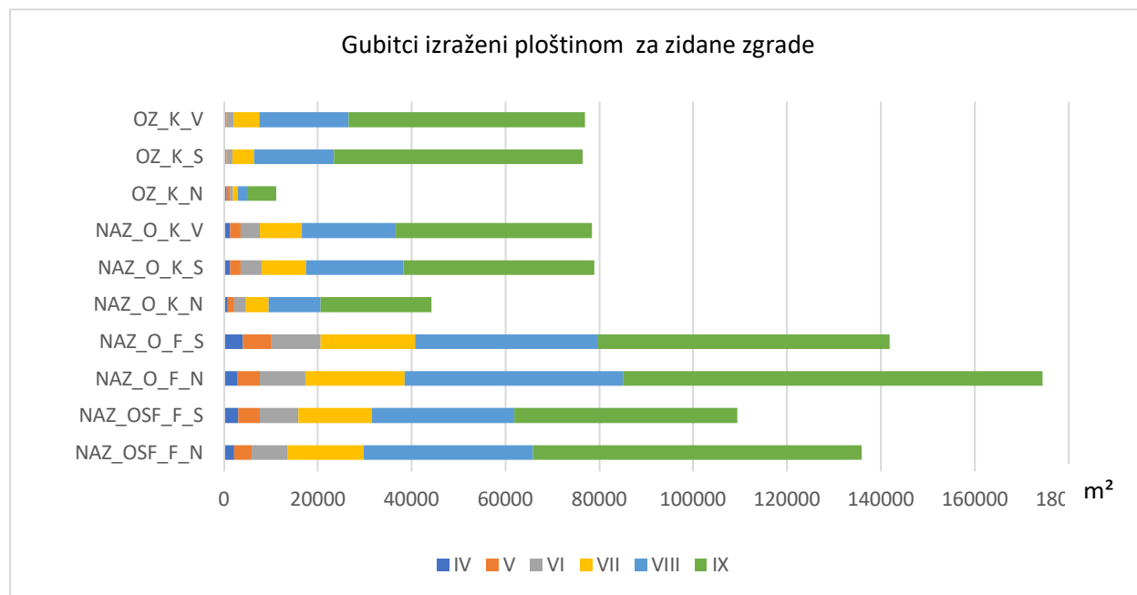
Slika 6.8 Gubitci za zidane zgrade iz modela izloženosti grada Osijeka, za stupnjeve intenziteta: IV., V., VI., VII., VIII. i IX. izražani ploštinom
