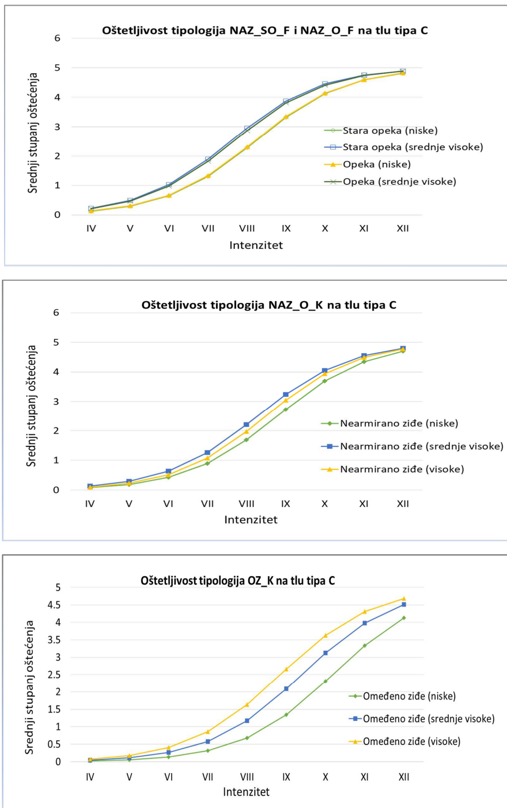
Slika 5.13 Srednji stupanj oštećenja tipologija zidanih zgrada
