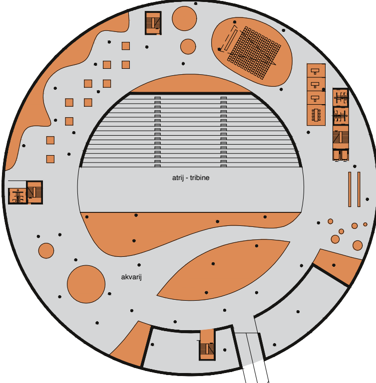
muzej podunavlja - tlocrt kata M 1:1000
