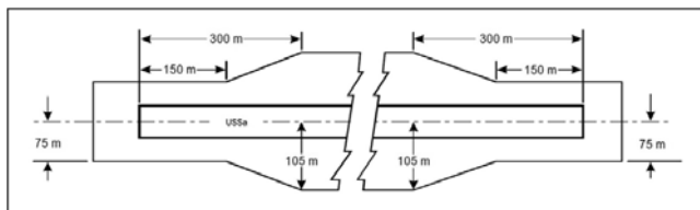
Slika A-4. Poravnati dio osnovne staze, uključujući uzletno-sletnu stazu za instrumentalno precizno prilaženje uzletno-sletnoj stazi kodnog broja 3 ili 4
