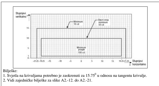
Slika A2.-14. Dijagram izokandela za svjetla središnje crte staze za vožnju (razmak 7.5 m) i svjetla stop-prečke u zakrivljenim sekcijama namijenjena korištenju u uvjetima kad je vidljivost manja od 350 m
