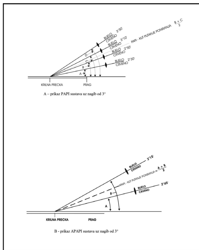
Slika 5-22 Nagib prilaza definiran za sustave PAPI i APAPI
