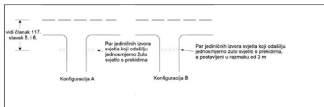
Slika 5-30. Sustav sigurnosnih svjetala uzletno-sletne staze
