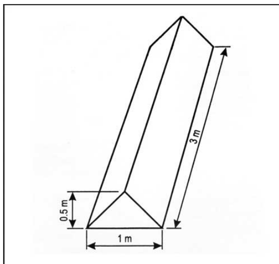
Slika 5-35. Označivač granice
