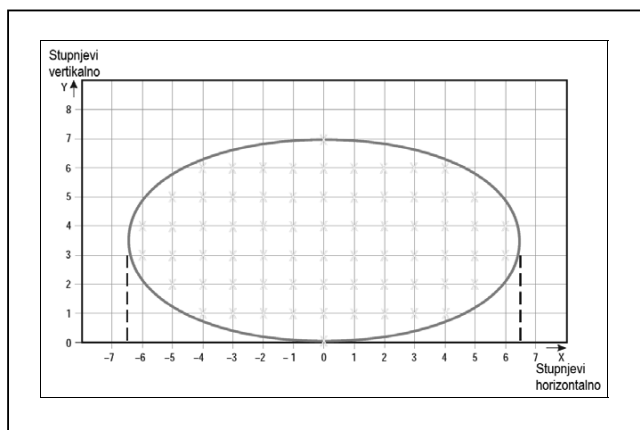
Slika A2.-11. Točke mreže koje se koriste za izračun prosječne jakosti svjetla sustava prilazne rasvjete i rasvjete uzletno-sletne staze
