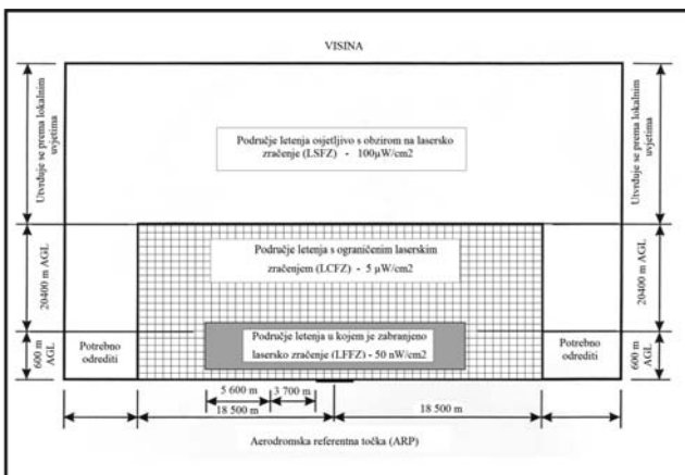
Slika 5-15. Zaštićena područja letenja s najvišim dozvoljenim vrijednostima isijavanja vidljivih laserskih zraka (AGL = iznad razine tla)
