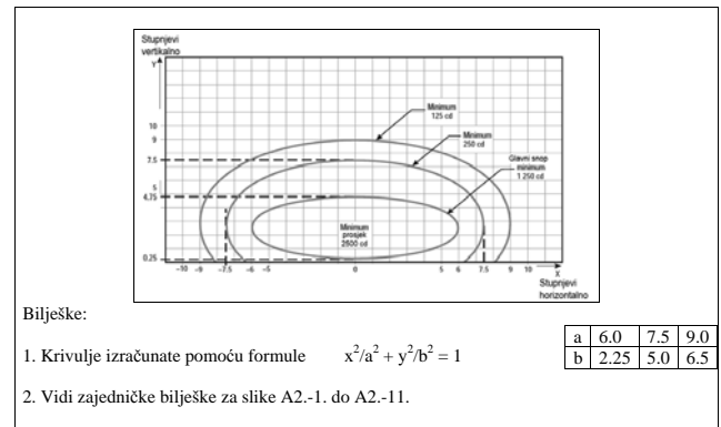
Slika A2-8. Dijagram izokandela za svjetla na kraju uzletno-sletne staze (crveno svjetlo)
