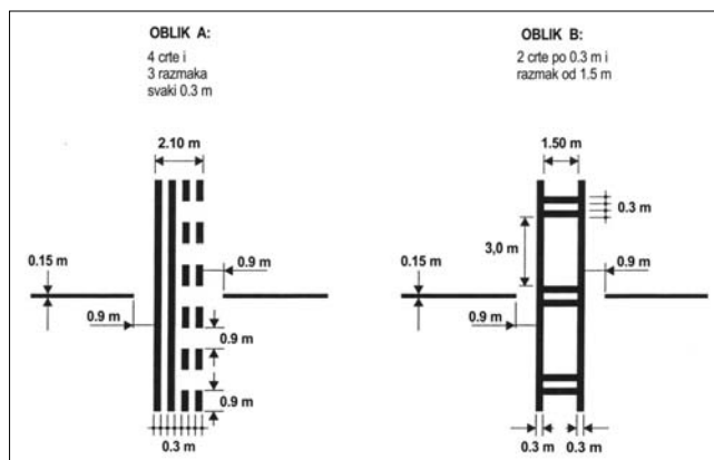
Slika 5.9. Oznake pozicije za čekanje
