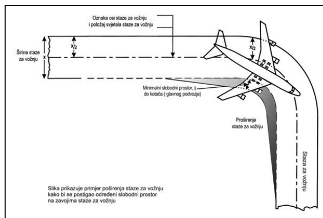
Slika 3 – 2. Zavoj na stazi za vožnju
