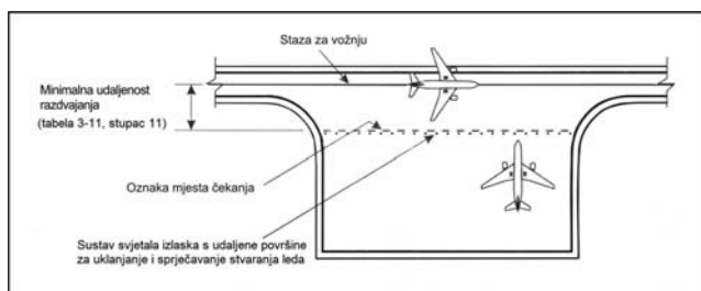
Slika 5-29. Tipična udaljena površina za uklanjanje i sprječavanje stvaranja leda
