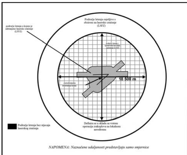
Slika 5-13. Područje letenja bez utjecaja laserskog zračenja
