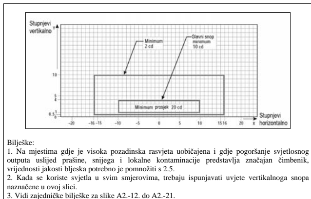
Slika A2.-15. Dijagram izokandela za svjetla središnje crte staze za vožnju (razmak 30 m, 60 m) i svjetla stop-prečke u ravnim sekcijama namijenjena korištenju u uvjetima kad je vidljivost minimalno 350 m
