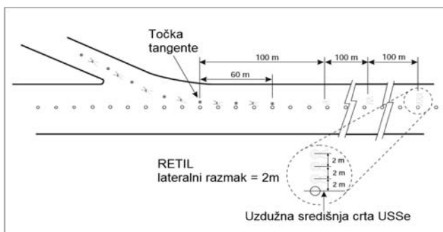
Slika 5-26. Svjetlosni pokazivači brzih izlaznih staza za vožnju
