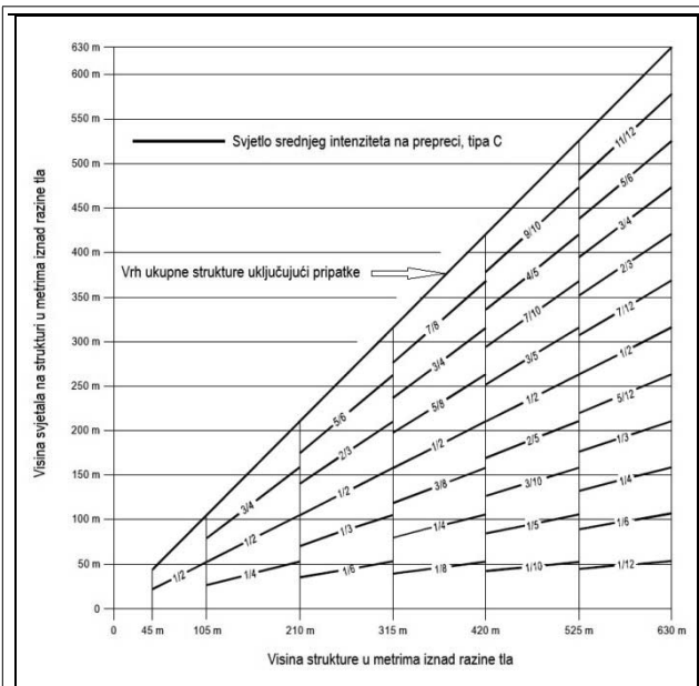
Bilješka. – Samo za korištenje noću. Slika A6.-3. Sustav jediničnih izvora svjetla koji odašilju svjetlost bez prekida, srednjeg intenziteta, crvene boje, tipa C, na preprekama
