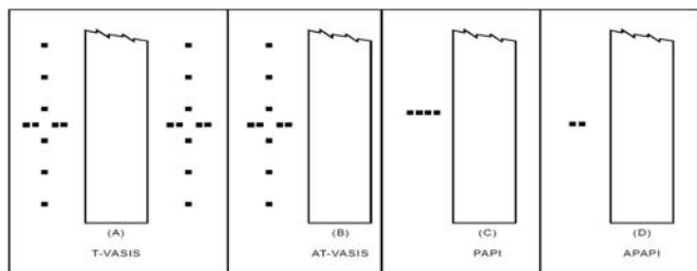
Slika 5-18. Sustavi svjetlosnih pokazivača nagiba prilaza
