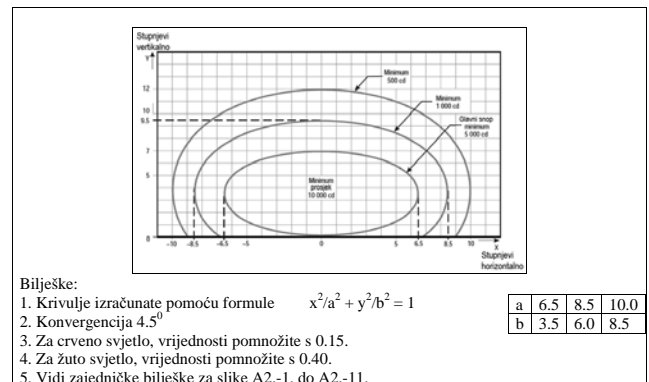
Slika A2-10. Dijagram izokandela za rubno svjetlo uzletno-sletne staze širine 60 (bijelo svjetlo)
