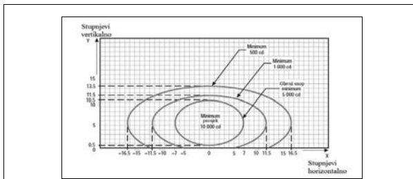
Slika A2-3. Dijagram izokandela za svjetlo praga (zeleno svjetlo)
