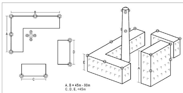
Slika 6-3. Osvjetljavanje zgrada
