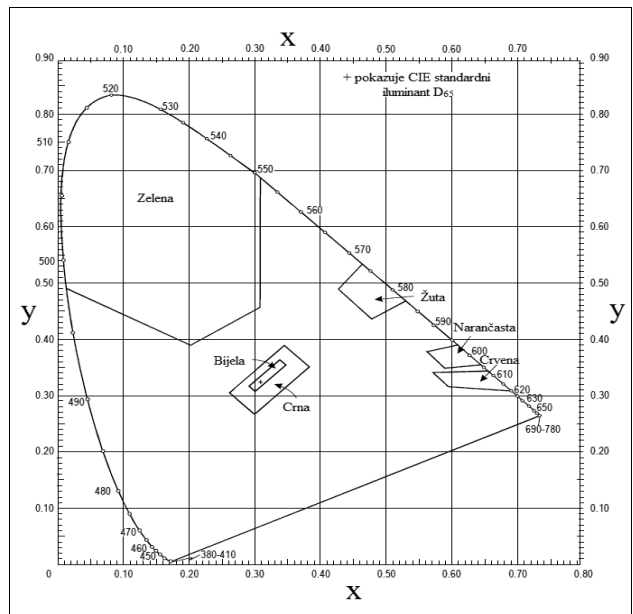
Slika A1-2. Obične boje za oznake i izvana osvijetljene znakove i ploče
