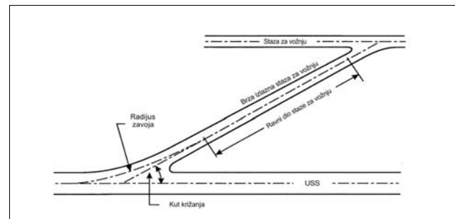
Slika 3-3. Brza izlazna staza za vožnju
