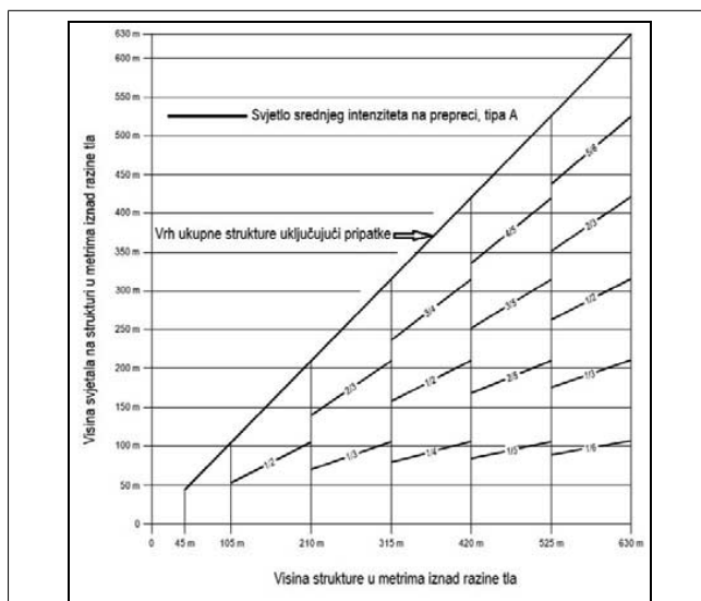
Bilješka. – Jedinični izvori svjetla visokog intenziteta na preprekama preporučeni su na strukturama visine veće od 150 m iznad razine tla. Ako se koriste jedinični izvori svjetla srednjeg intenziteta, potrebne su također oznake.
