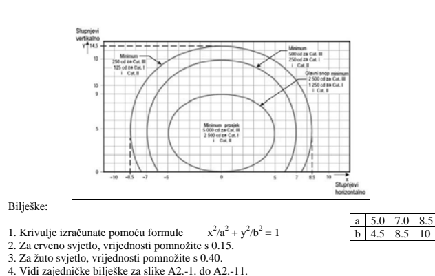
Slika A2-7. Dijagram izokandela za svjetlo središnje crte USSE longitudinalnog razmaka 15 m (bijelo svjetlo) i kratkog svjetla pokazatelja izlazne staze za vožnju (žuto svjetlo)
