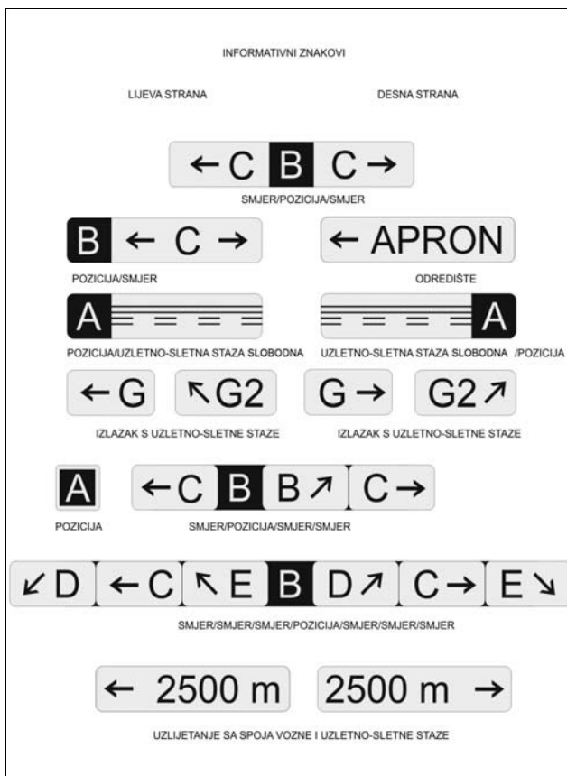
Slika 5-32. Informativni znakovi
