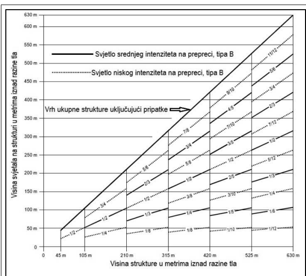
Bilješka. – Samo za korištenje noću. Slika A6.-2. Sustav crvenih treptajućih svjetala srednjeg intenziteta, tipa B, na preprekama
