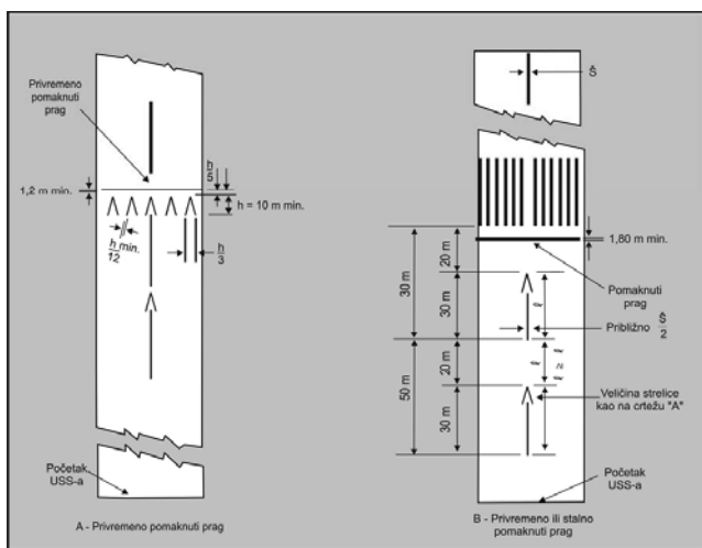
Slika 5-4. Oznake pomaknutog praga
