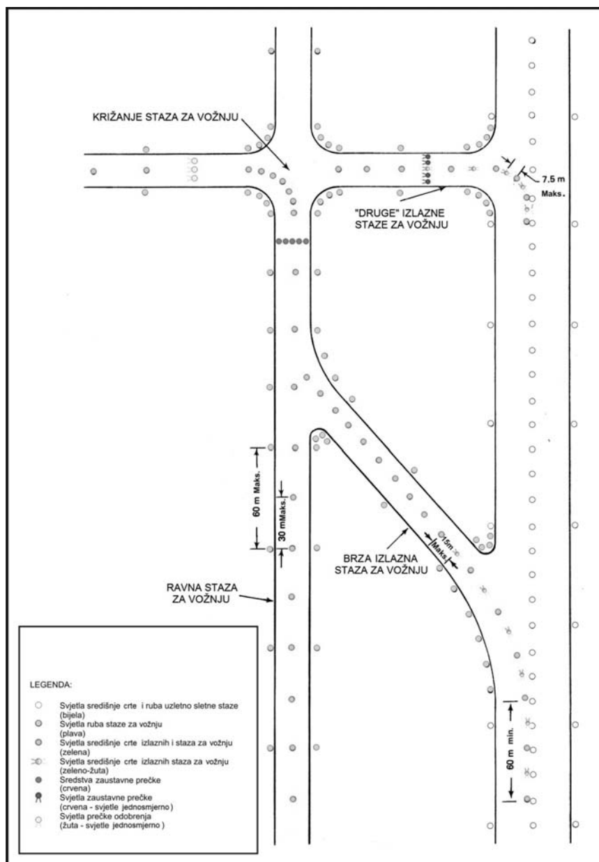
Slika 5-27 Sustavi svjetala staze za vožnju
