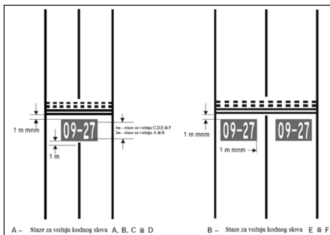
Slika 5-12. Oznake naredaba
