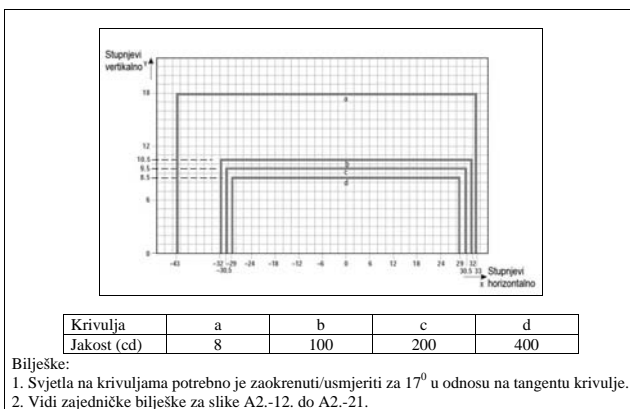
Slika A2.-19. Dijagram izokandela za svjetla središnje crte staze za vožnju velike jakosti (razmak 7.5 m) i svjetla stop-prečke u zakrivljenim sekcijama namijenjena korištenju u naprednom sustavu za navođenje i kontrolu površinskog kretanja u slučajevima kada su potrebna svjetla veće jakosti
