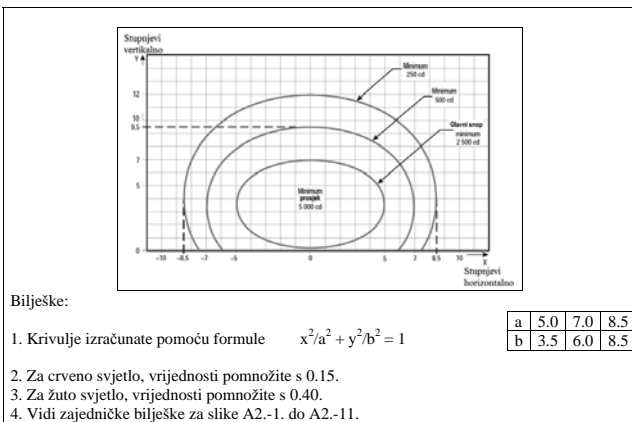
Slika A2-6. Dijagram izokandela za svjetlo središnje linije USSE longitudinalnog razmaka 30 m (bijelo svjetlo) i kratkog svjetla pokazatelja izlazne rulne staze (žuto svjetlo)
