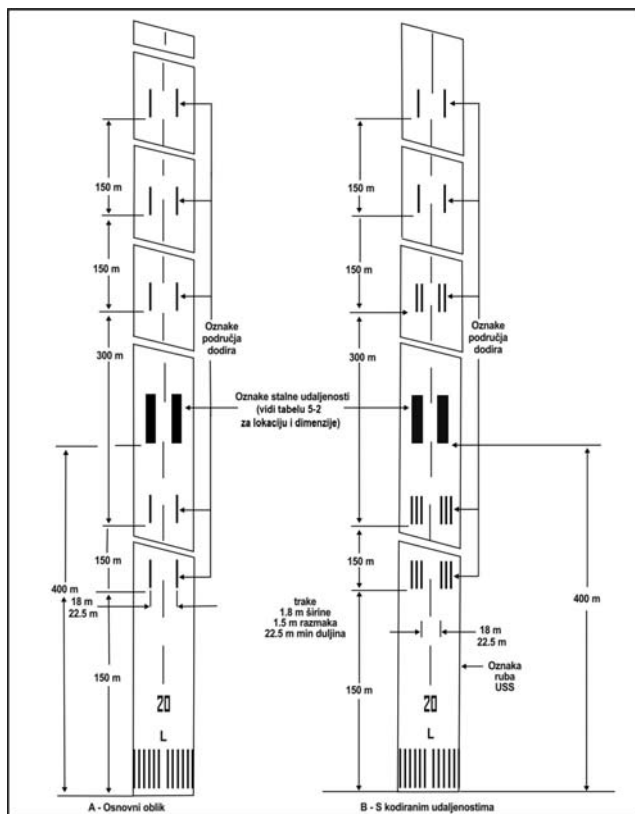
Slika 5-5. Oznake ciljne točke i područja dodira na uzletno-sletnoj stazi duljine \geq 200 m
