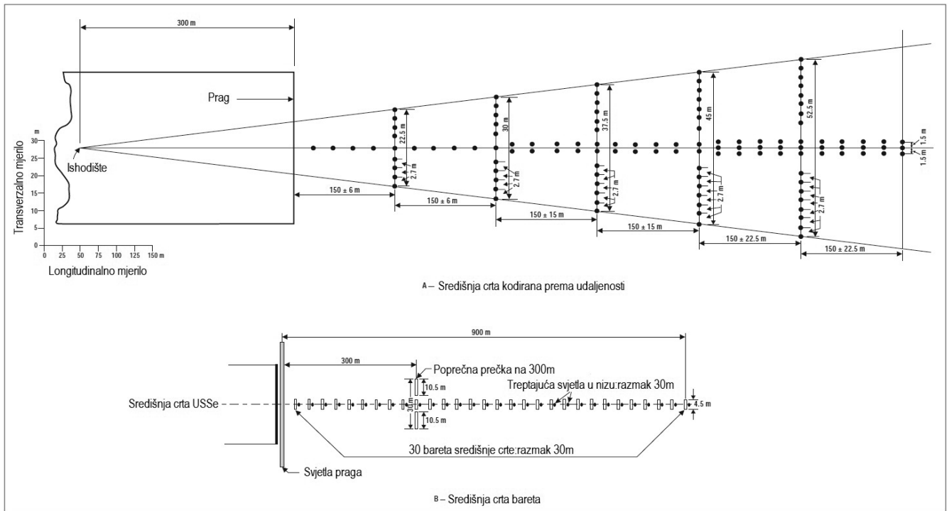
Slika A-7. Sustavi prilazne rasvjete za instrumentalni precizni prilaz kategorije I
