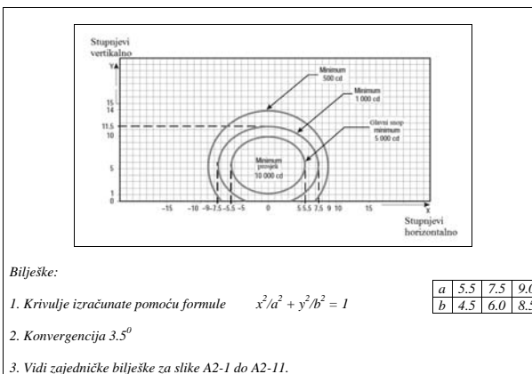
Slika A2-3. Dijagram izokandela za svjetlo praga (zeleno svjetlo)
