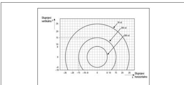
Slika A2.-23. Distribucija jakosti svjetla PAPI-a i APAPI-a
