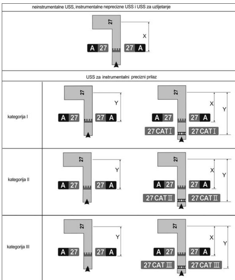
Slika 5-33. Primjeri položaja znakova na križanjima staze za vožnju i uzletno-sletne staze
