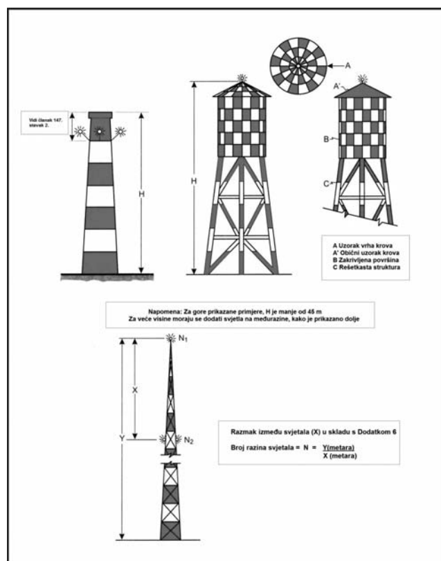
Slika 6-2. Primjeri označavanja i osvijetljavanja visokih objekata
