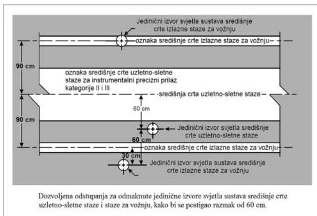
Slika 5-28. Odmaknuti jedinični izvori svjetla sustava svjetala središnje crte uzletno-sletne staze i staze za vožnju
