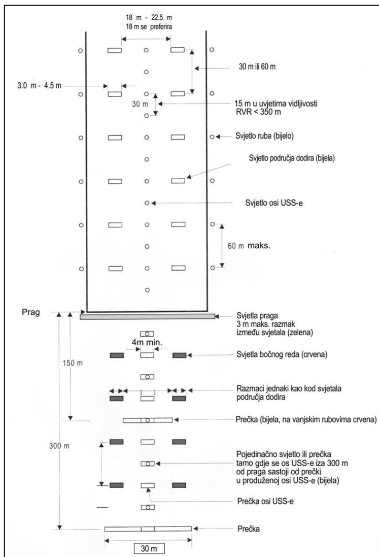
Slika 5-17. Unutarnjih 300 m sustava prilazne rasvjete i sustava rasvjete uzletno-sletne staze za instrumentalni precizni prilaz kategorije II ili III, ukoliko operator aerodroma osigura ispravnost sustava prilazne rasvjete definiran u članku 189. stavku 8. ovoga Pravilnika
