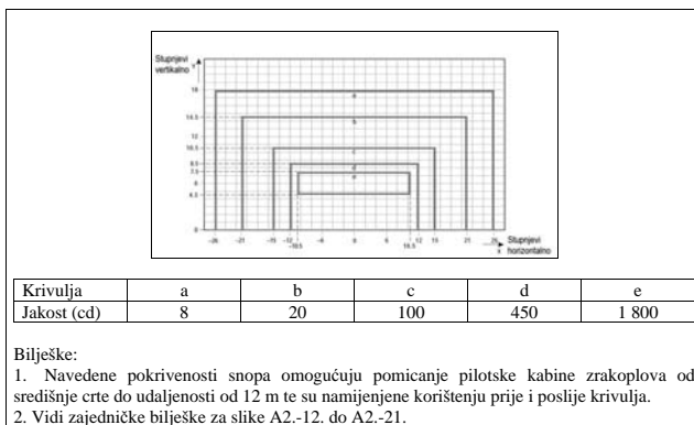
Slika A2.-17. Dijagram izokandela za svjetla središnje crte staze za vožnju velike jakosti (razmak 15 m) i svjetla stop-prečke u ravnim sekcijama namijenjena korištenju u naprednom sustavu za navođenje i kontrolu površinskog kretanja u slučajevima kada su potrebna svjetla veće jakosti i kada može doći do velikih suprotnih djelovanja
