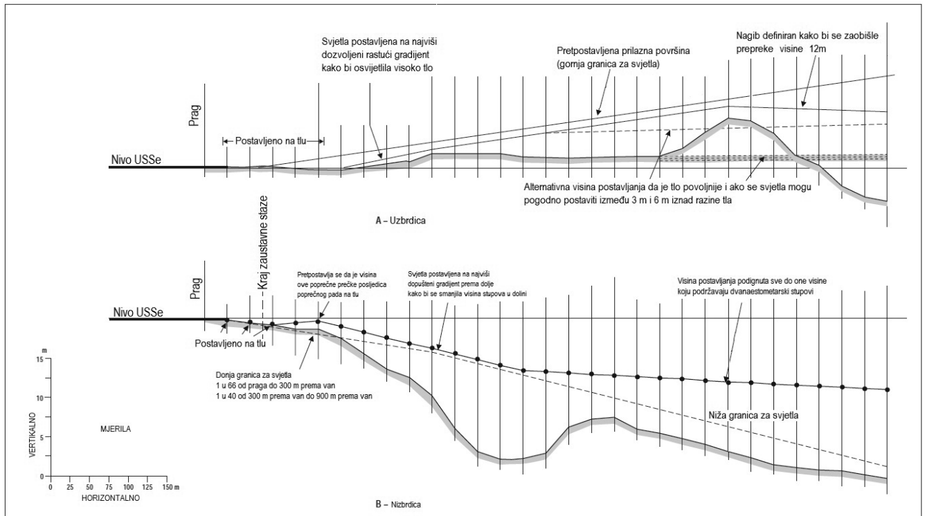
Slika A-8. Okomito dopušteno odstupanje instaliranja
