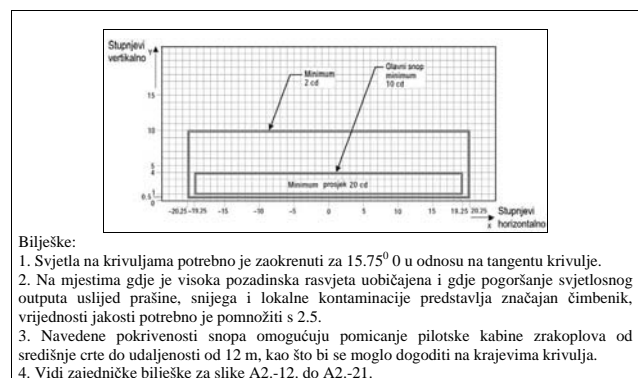
Slika A2.-16. Dijagram izokandela za svjetla središnje crte staze za vožnju (razmak 7.5 m, 15 m, 30 m) i svjetla stop-prečke u zakrivljenim sekcijama namijenjena korištenju u uvjetima kad je vidljivost minimalno 350 m
