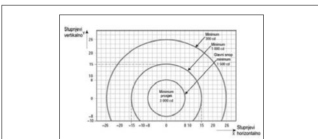
Slika A2.-24. Dijagram izokandela za svaki jedinični izvor u sustavu sigurnosnih svjetala uzletno-sletne staze male jakosti, konfiguracija A
