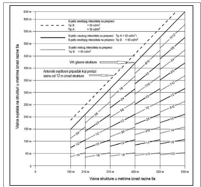
Slika A6-7. Dualni sustav rasvjete prepreka visokog/srednjeg intenziteta, tipa A/tipa B
