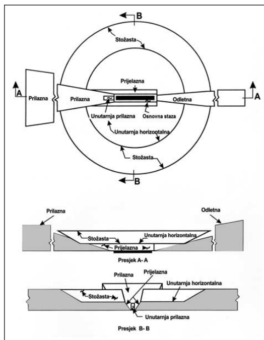
Slika 4-1 Površine ograničenja prepreka
