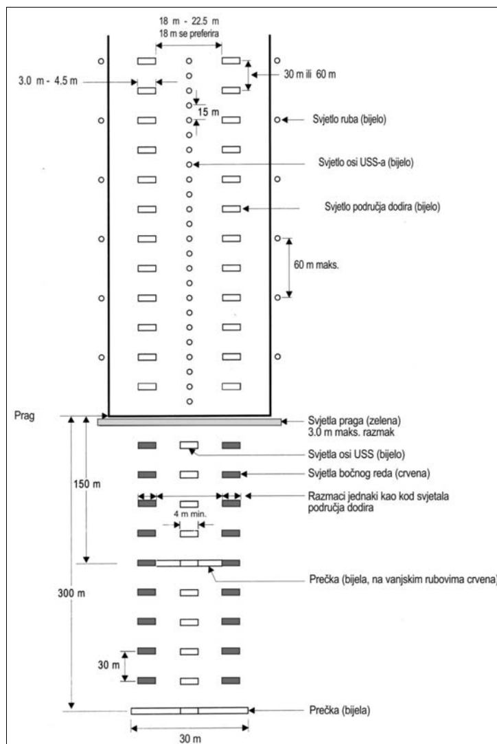
Slika 5-16. Unutarnjih 300 m svjetala prilaza i svjetala uzletno-sletne staze kod uzletno-sletnih staza za precizni prilaz kategorije II ili III
