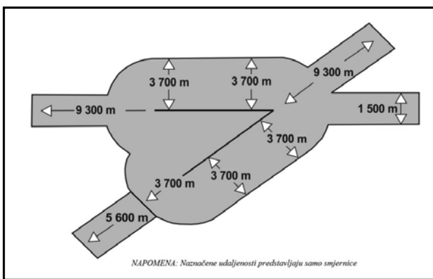
Slika 5-14. Područje letenja bez utjecaja laserskog zračenja na primjeru dviju uzletno-sletnih staza
