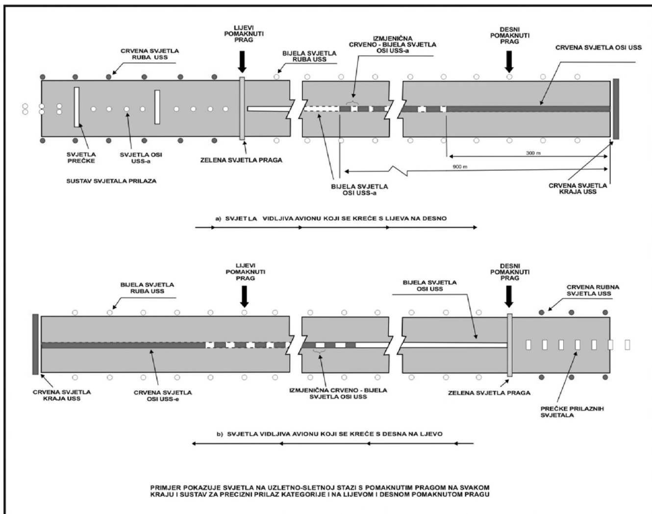
Slika 5-25. Primjer prilazne rasvjete i rasvjete uzletno-sletne staze s pomaknutim pragom
