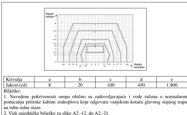
Slika A2.-18. Dijagram izokandela za svjetla središnje crte staze za vožnju velike jakosti (razmak 15 m) i svjetla stop-prečke u ravnim sekcijama namijenjena korištenju u naprednom sustavu za navođenje i kontrolu površinskog kretanja u slučajevima kada su potrebna svjetla veće jakosti
