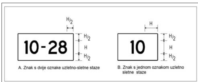
Slika A4.-3. Dimenzije znakova
