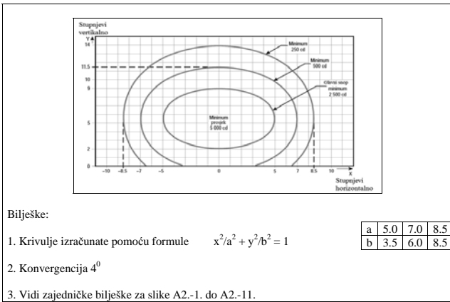
Slika A2-5. Dijagram izokandela za svjetlo područja dodira (bijelo svjetlo)
