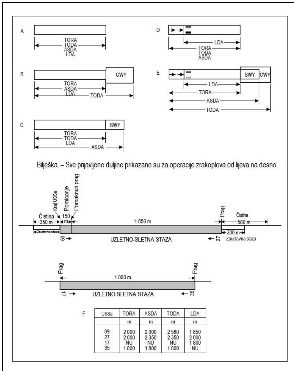
Slika A-1. Prikaz objavljenih duljina
