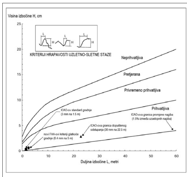
Slika A-3. Usporedba kriterija hrapavosti
