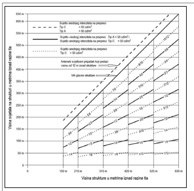
Slika A6.-8. Dualni sustav rasvjete prepreka visokog/srednjeg intenziteta, tipa A/tipa C
