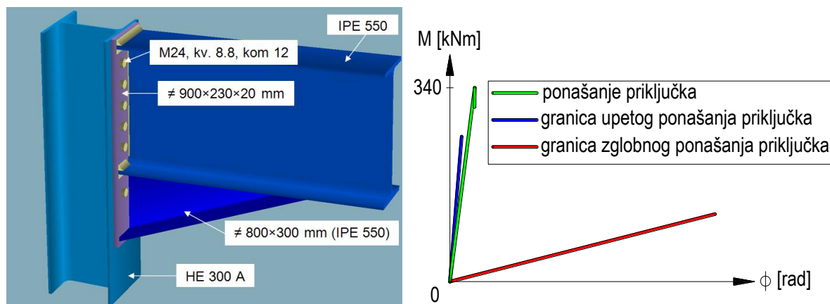
Slika 6 - Suvremeno rješenje priključka prečke i stupa s pripadajućim M_i - \phi dijagramom (1. varijanta)
