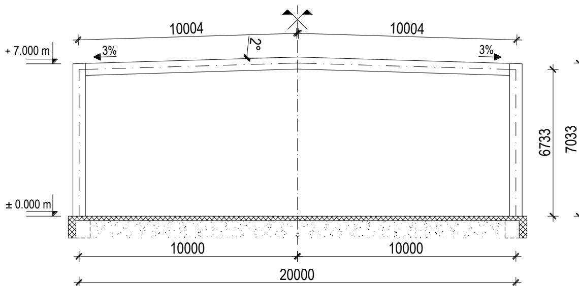
Slika 4 - Razmatrani dvozglobni okvir
