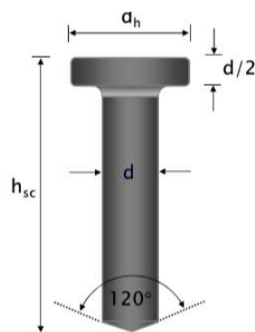
Slika 8.3 – Moždanik s glavom
