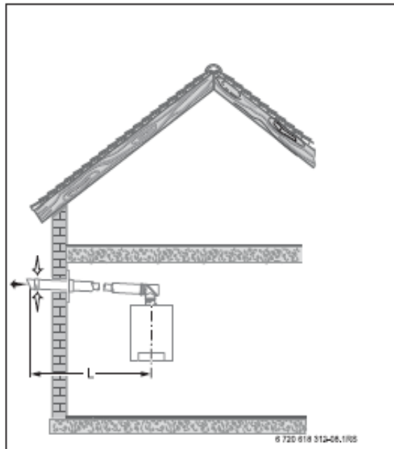
Slika 45 C 13 : Dovod zraka/odvod dimnih plinova kroz koncentričnu cijev Ø 100/150 mm, horizontalno kroz pročelje
