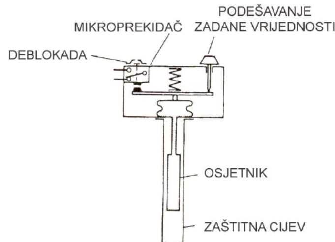
Dvopoložajni regulator
