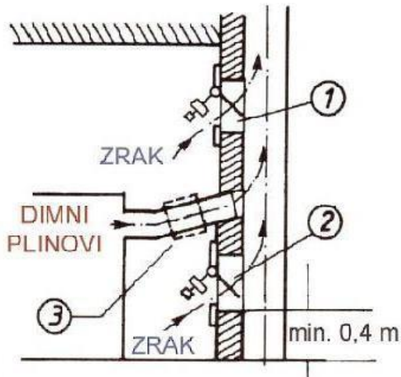
Primjeri ugradnje graničnika propuha
