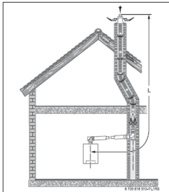
Slika 48 C 33 : Dovod zraka/odvod dimnih plinova u dimovodnom oknu, kroz savitljivu cijev \varnothing 100 mm i u protustruji
