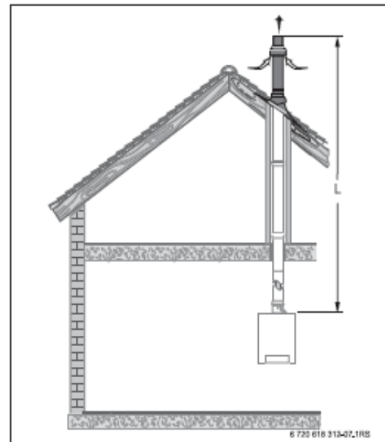
Slika 47 C 33 : Dovod zraka/odvod dimnih plinova kroz koncentričnu cijev Ø 100/150 mm, vertikalno iznad krova
