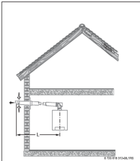
Slika 46 C 13 : Dovod zraka/odvod dimnih plinova kroz koncentričnu cijev Ø 100/150 mm, horizontalno kroz pročelje
