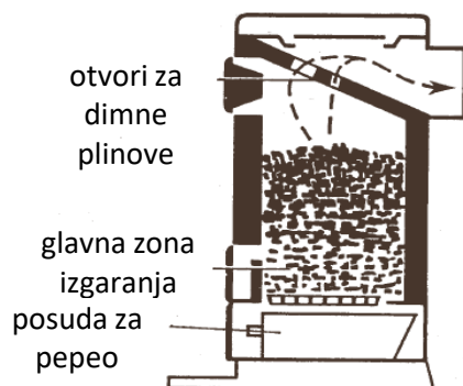
Željezna trajnožareća peć s progorijevanjem
