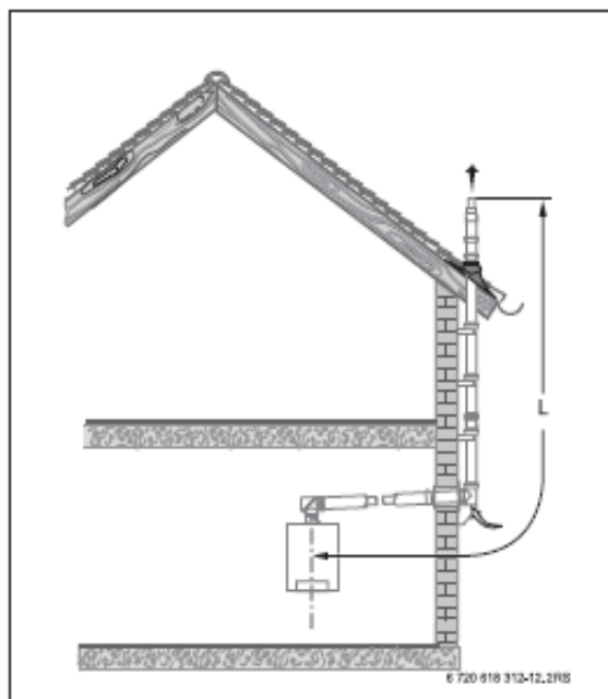
Slika 50 C 33 : Dovod zraka/odvod dimnih plinova kroz koncentričnu cijev \varnothing 100/150 mm, na pročelju
