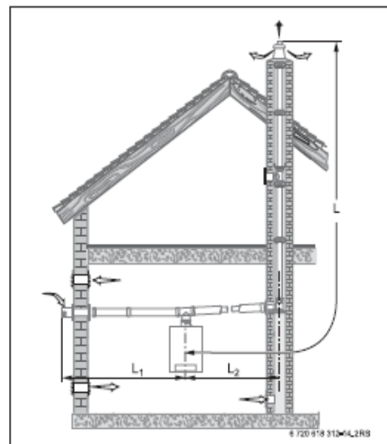
Slika 51 C 33 : Odvod dimnih plinova u dimovodnom oknu \varnothing 100 mm, vođenje zraka na pročelju
