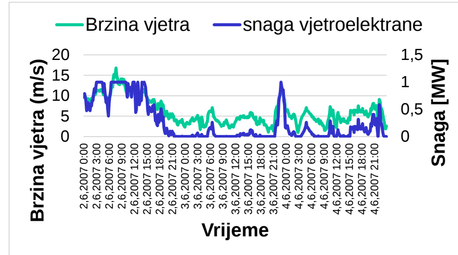
10-min mjerenja brzine vjetra (3 dana) i snaga VE
