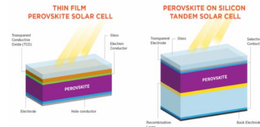
Perovskit
