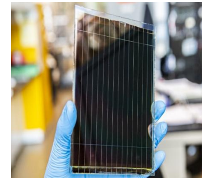
Perovskit
